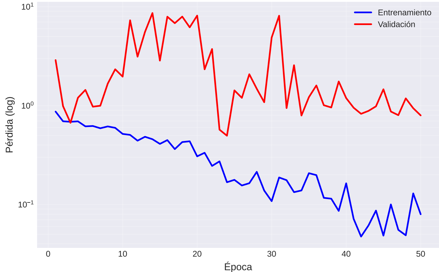
Pérdida en escala logarítmica
