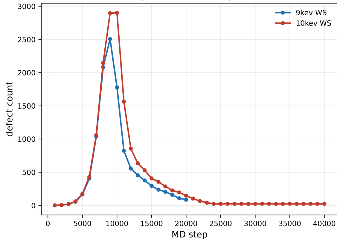
Wigner-Seitz Frenkel pairs
