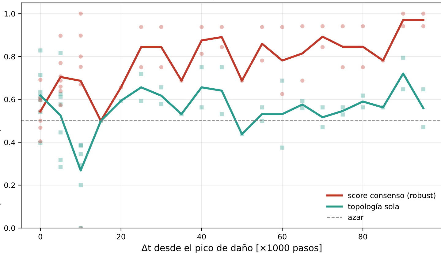
Horizonte de predictibilidad del daño superviviente (cascadas FeCrNi 4-8 keV; puntos = cascadas, línea = media)
