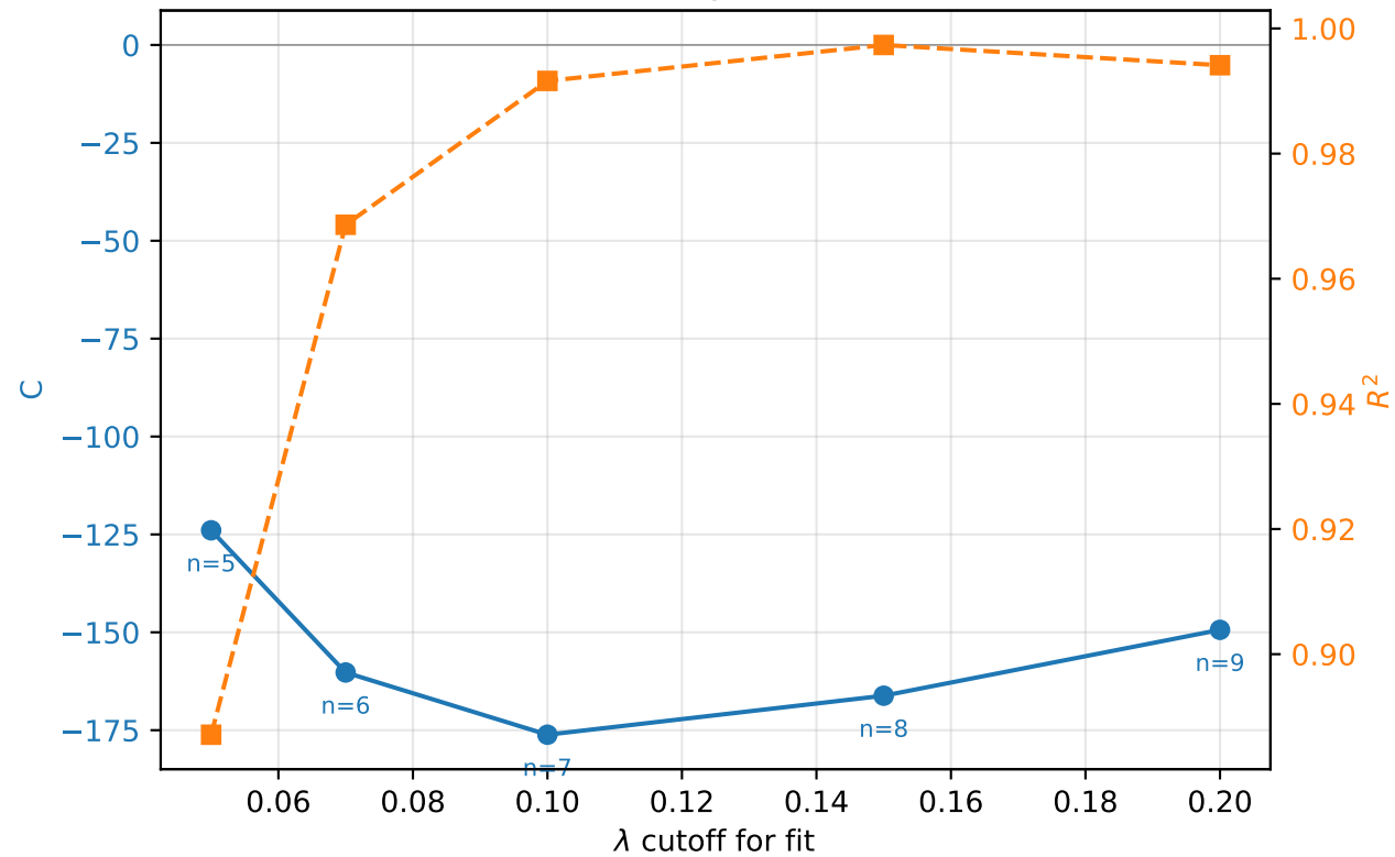
(d) C-fit stability across cutoffs
