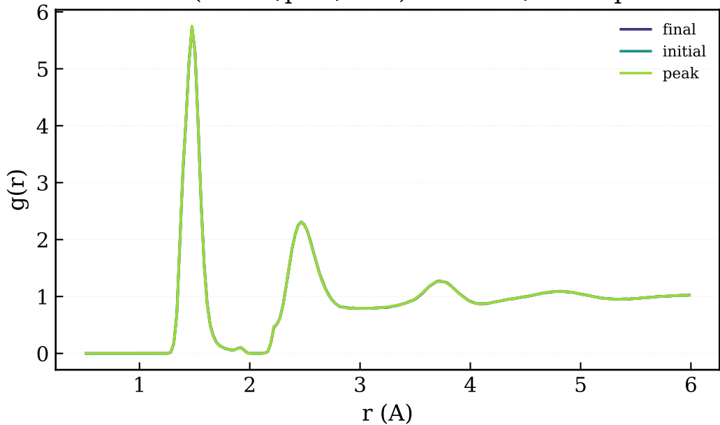
RDF (inicial/pico/final) - 10 keV / 20% sp3
