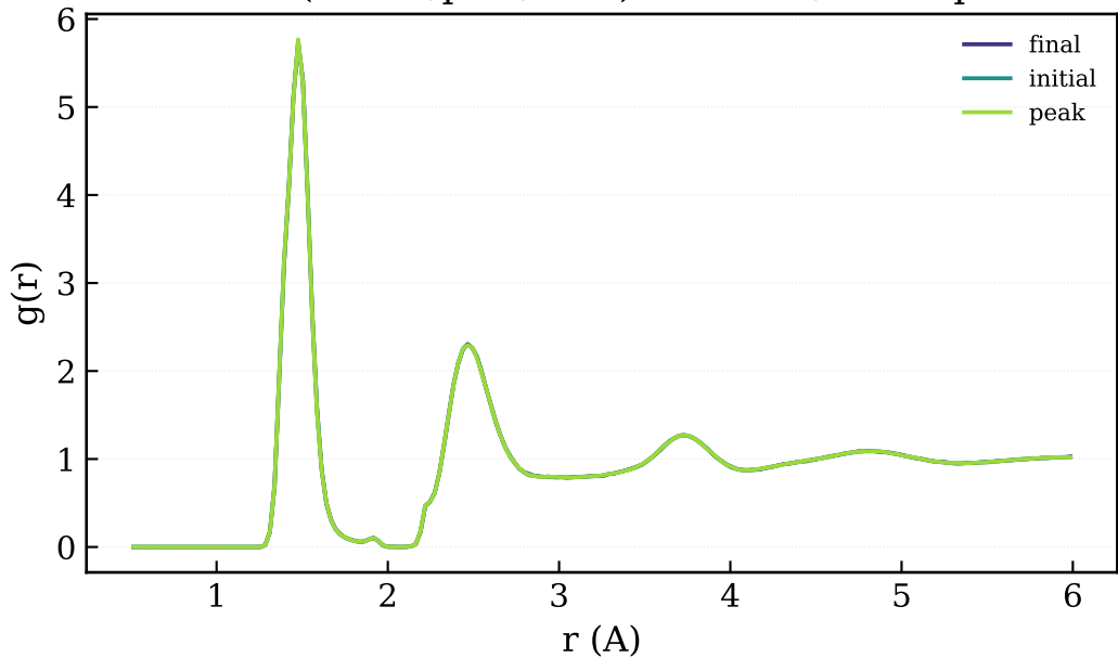
RDF (inicial/pico/final) - 15 keV / 20% sp3
