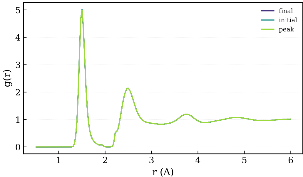
RDF (inicial/pico/final) - 15 keV / 40% sp3
