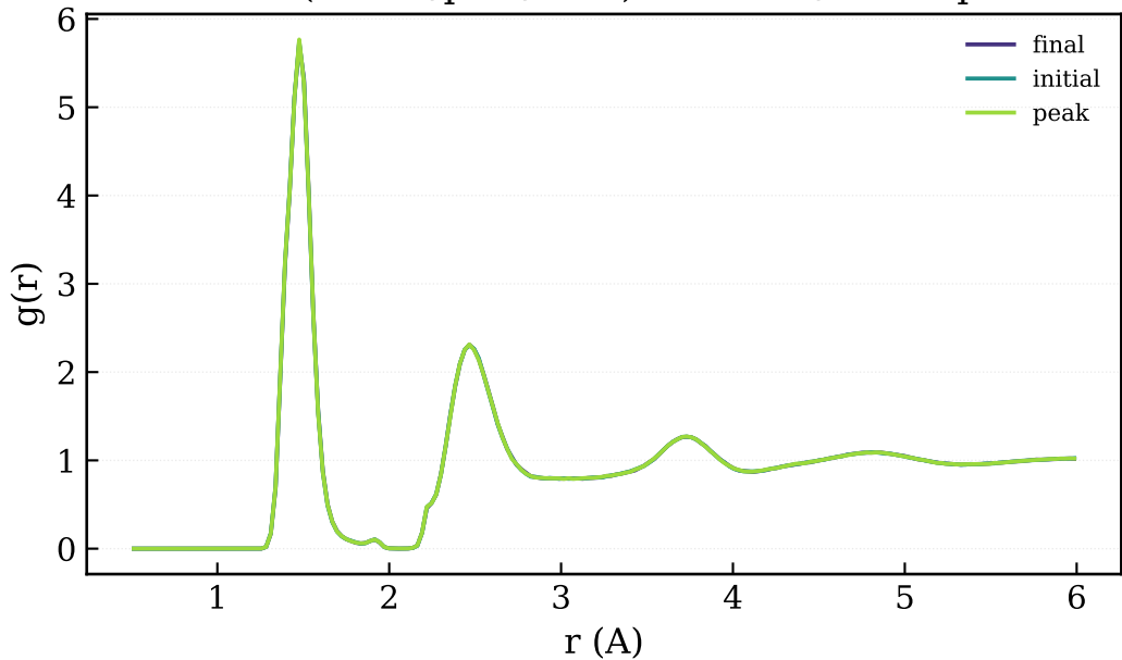
RDF (inicial/pico/final) - 20 keV / 20% sp3
