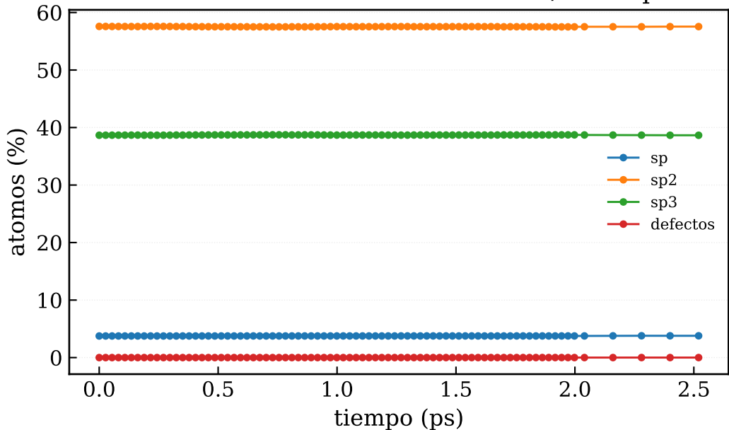
Evolucion de hibridacion - 20 keV / 40% sp3
