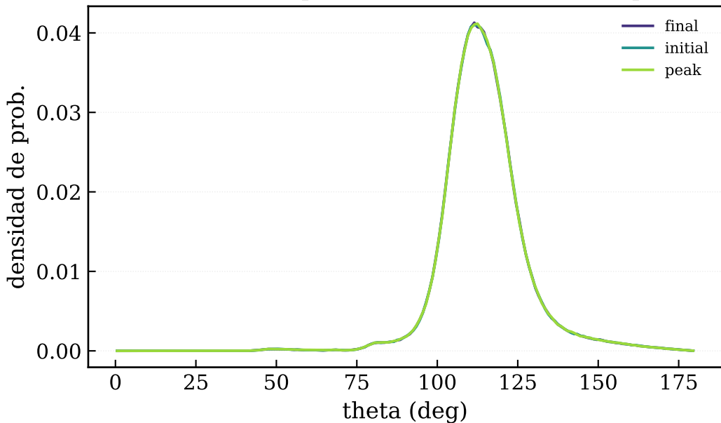
ADF (inicial/pico/final) - 25 keV / 20% sp3
