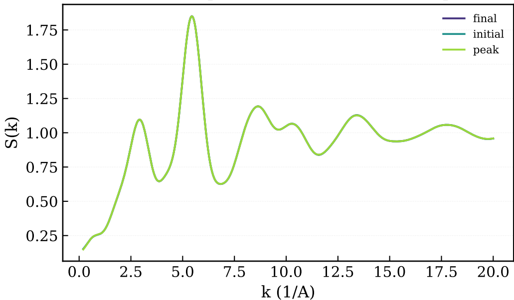
SK (inicial/pico/final) - 25 keV / 40% sp3
