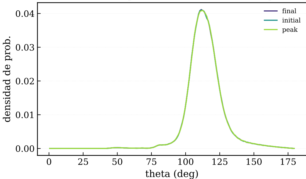
ADF (inicial/pico/final) - 30 keV / 20% sp3
