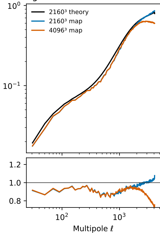
Segment 23: 0.174 < z < 0.211
