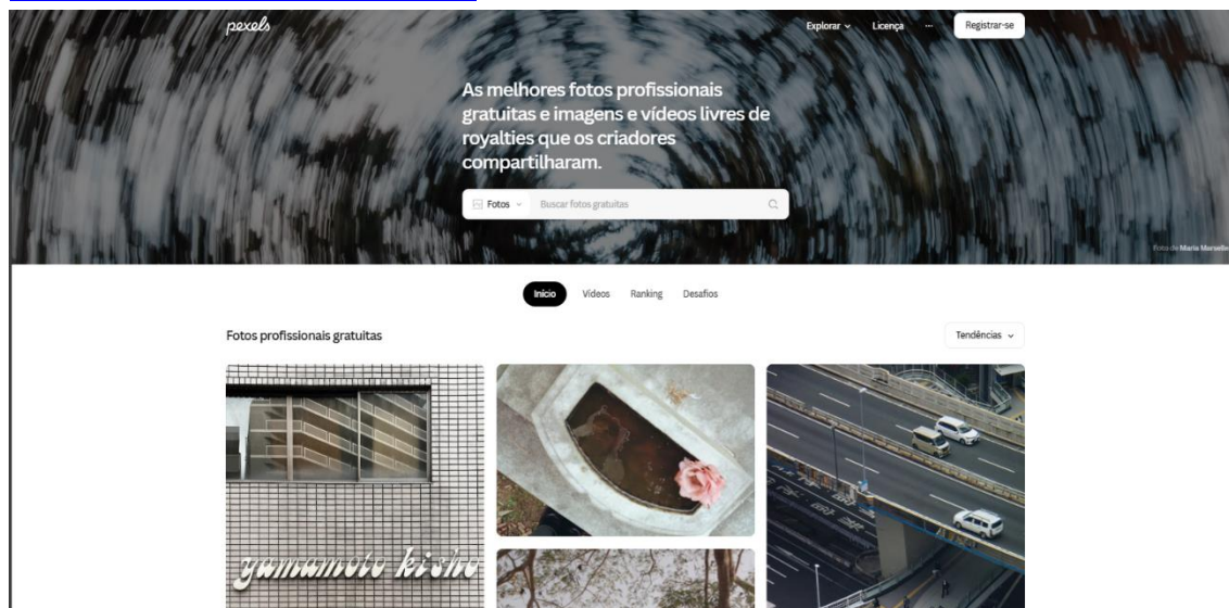
Figura 43-site2
