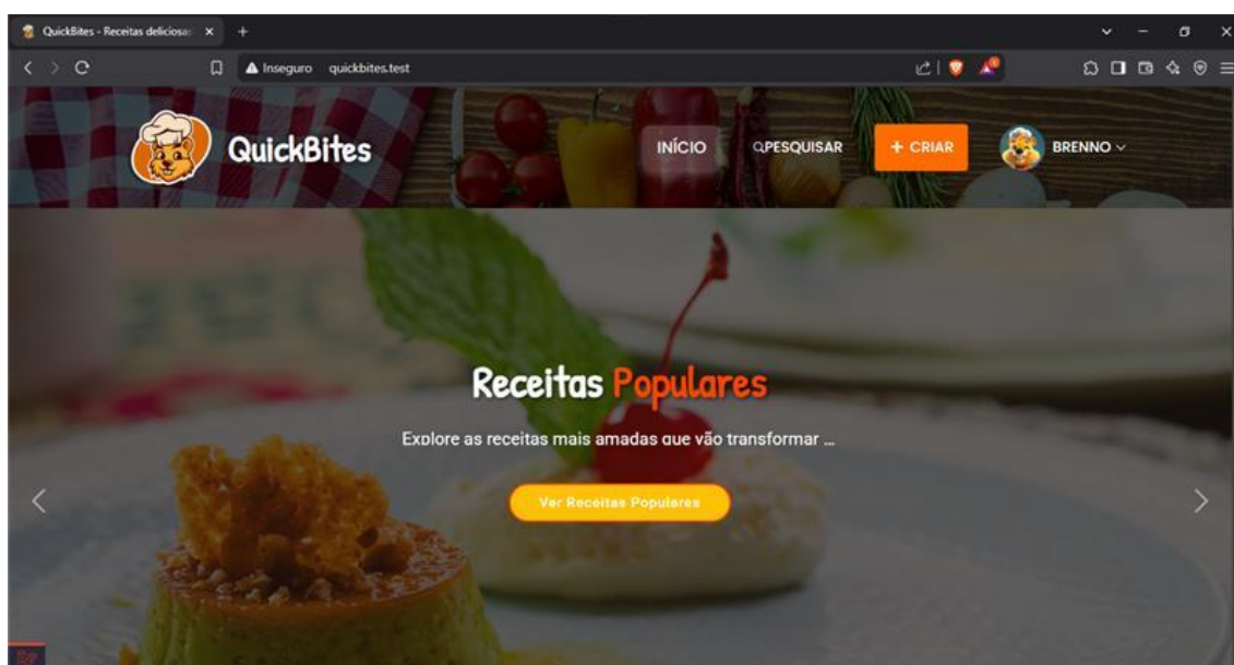
Figura 14-Home1
