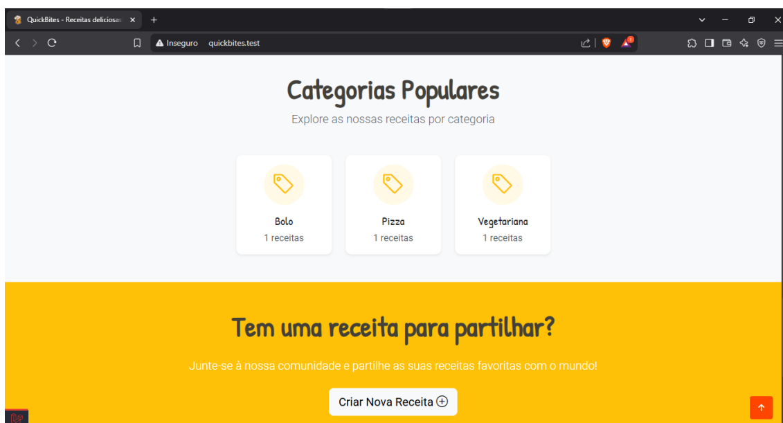
Figura 16-home3
