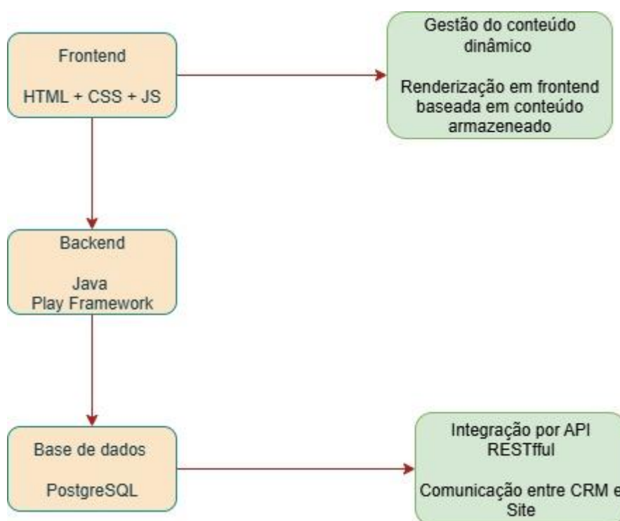
Figura 6 - Arquitetura do Sistema
