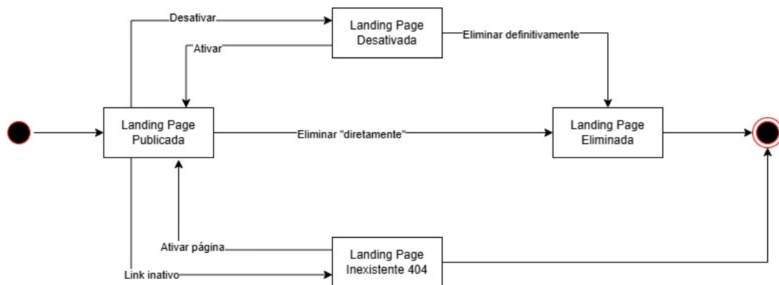
Figura 4 - Diagrama de estados
