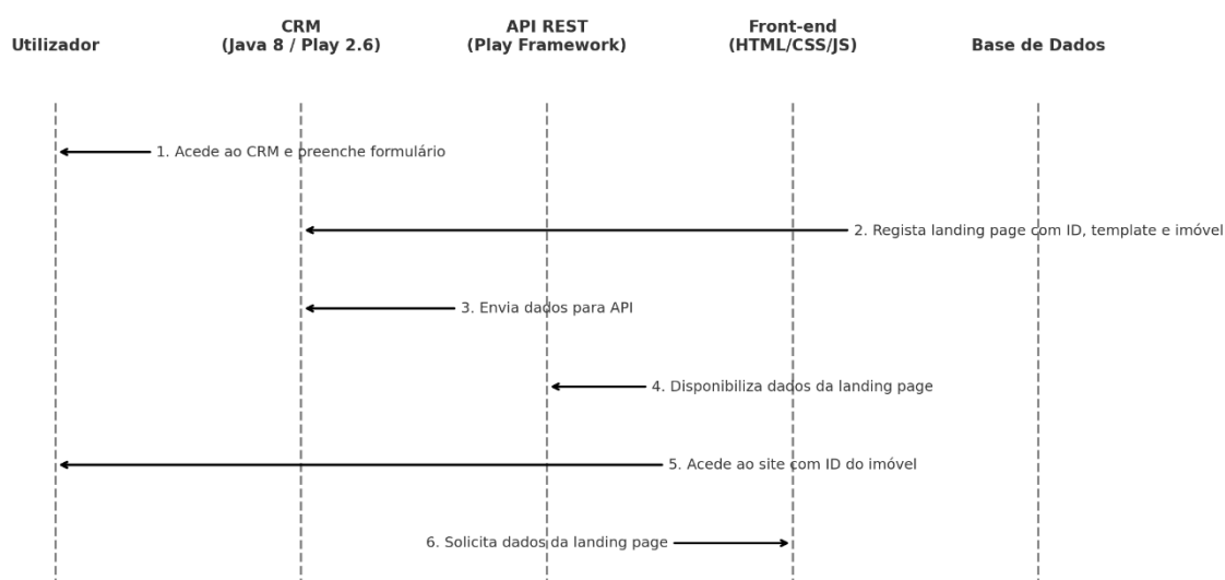
Figura 3 - Diagrama de Sequência
