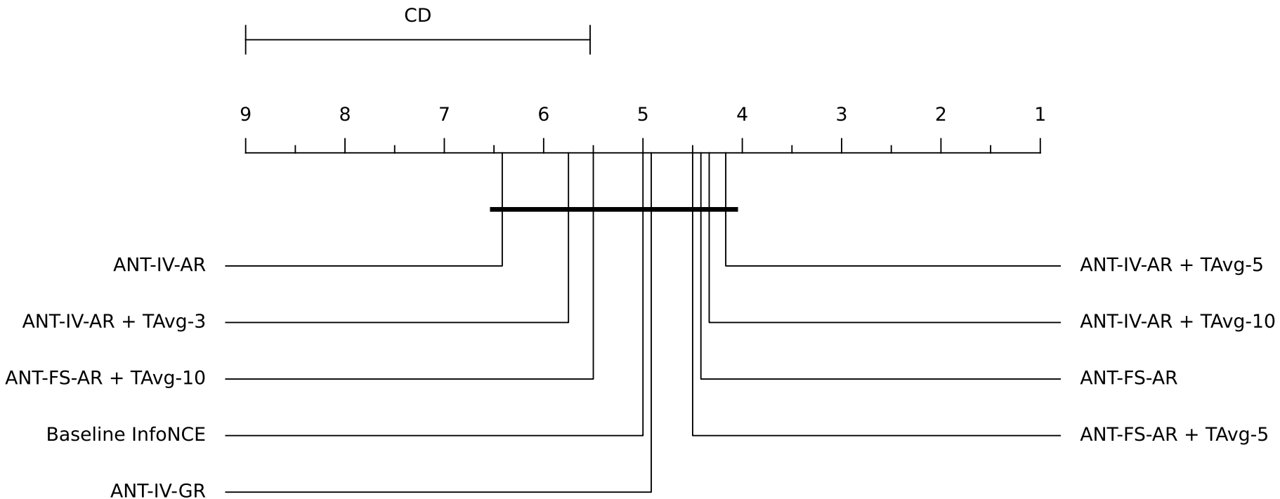
Diagrama de diferença crítica — AvgAcc 9 métodos × 12 blocos pareados | \alpha=0.05
