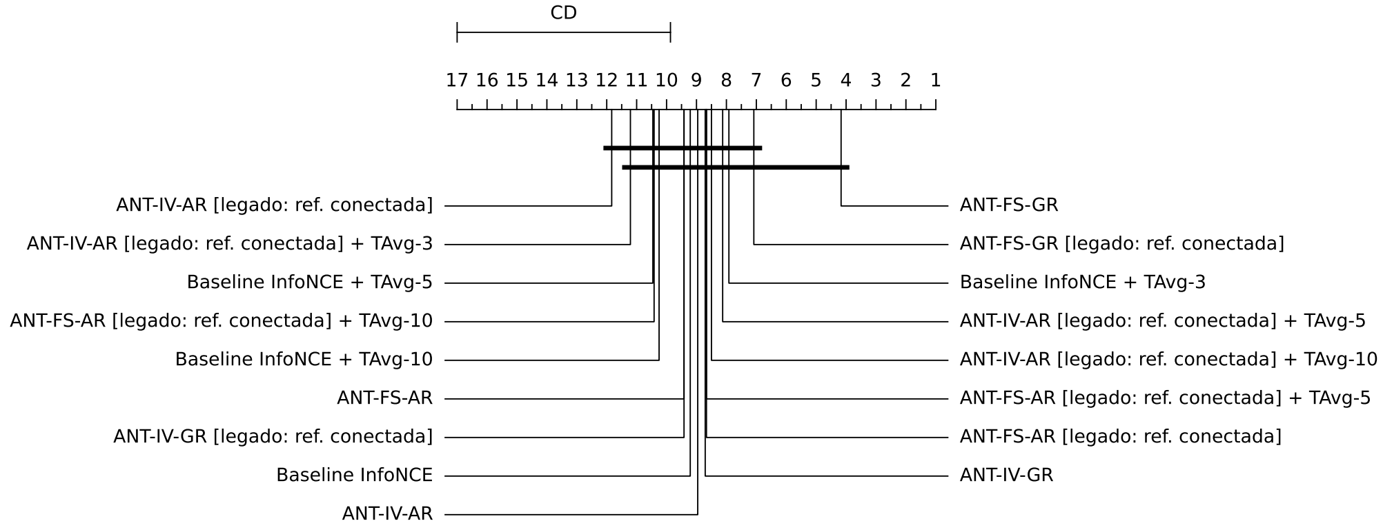
Diagrama de diferença crítica — AvgAcc 17 métodos × 12 blocos pareados | \alpha=0.05
