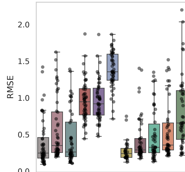
Dataset: Burkhardt
