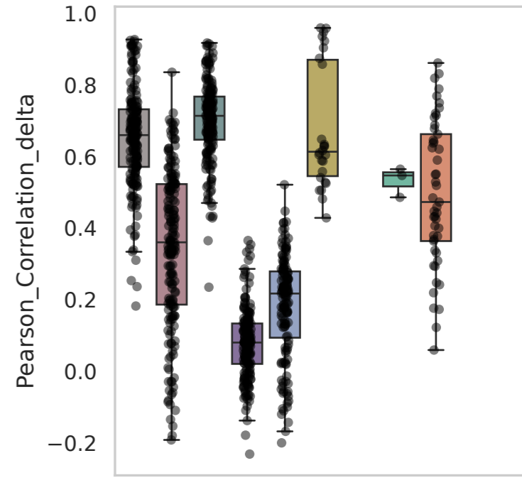
Dataset: Parse
