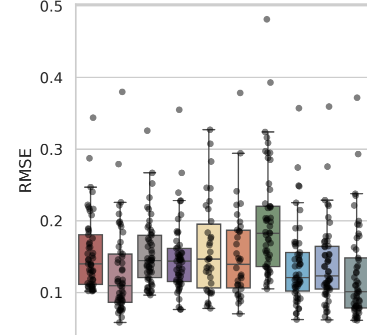
Dataset: Frangieh
