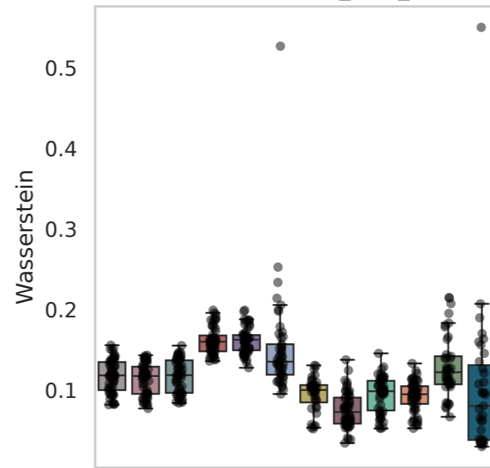
Dataset: Perturb_cmo_V1
