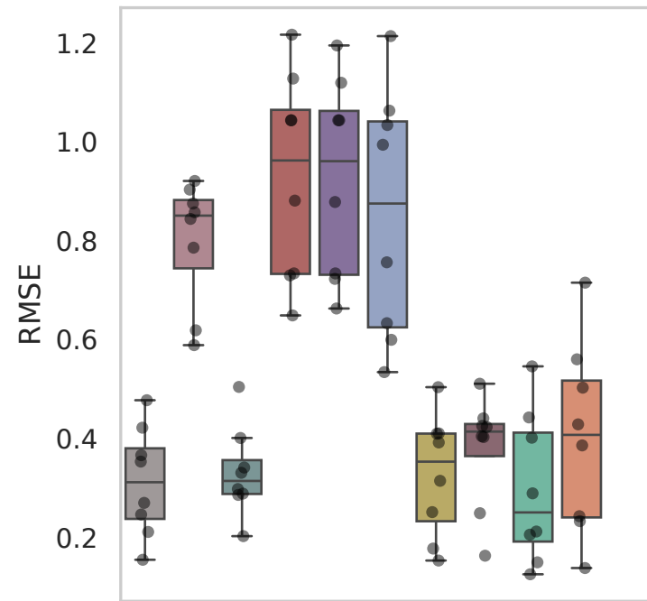
Dataset: Haber
