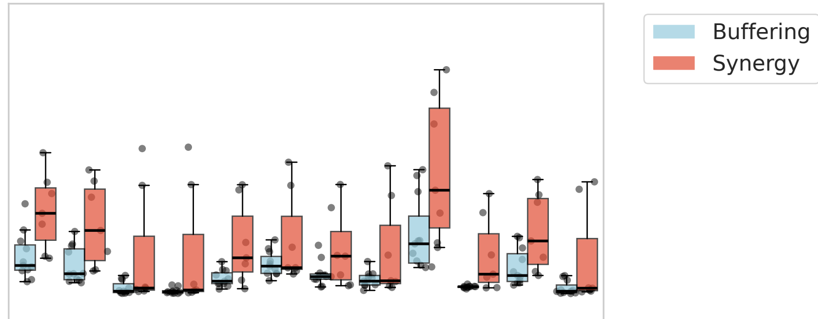
Seen2 Top20
