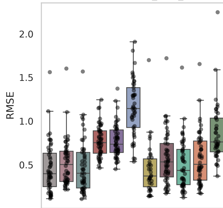
Dataset: Perturb_cmo_V1
