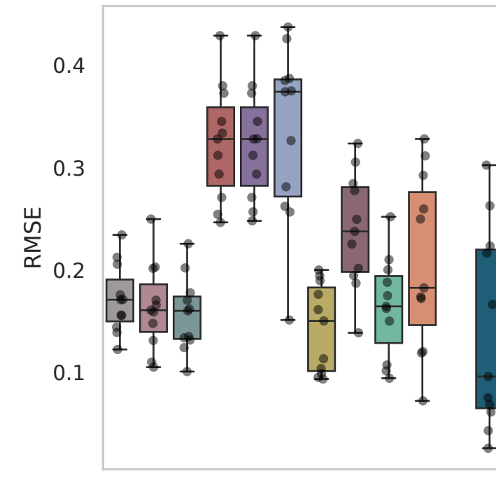
Dataset: Weinreb
