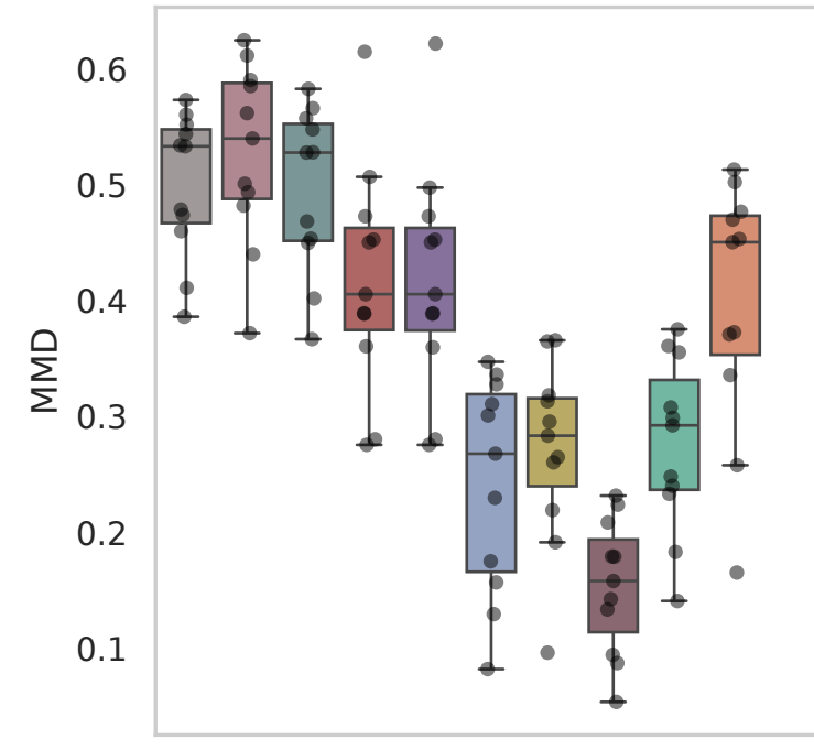
Dataset: Weinreb
