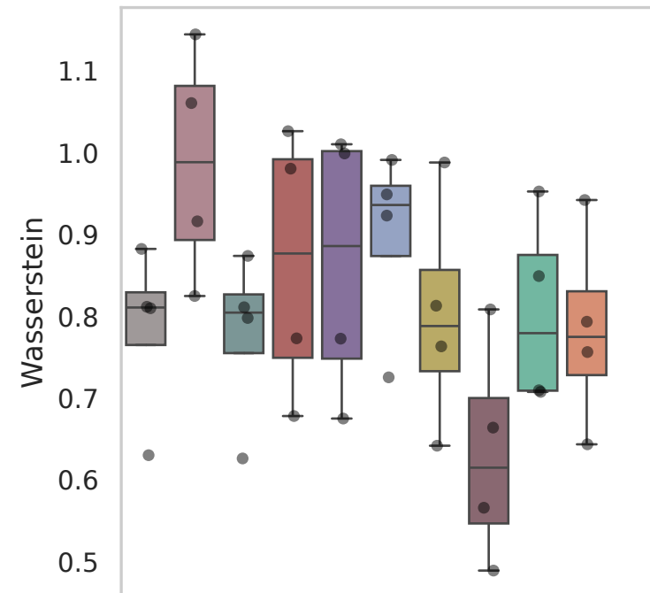
Dataset: Hagai
