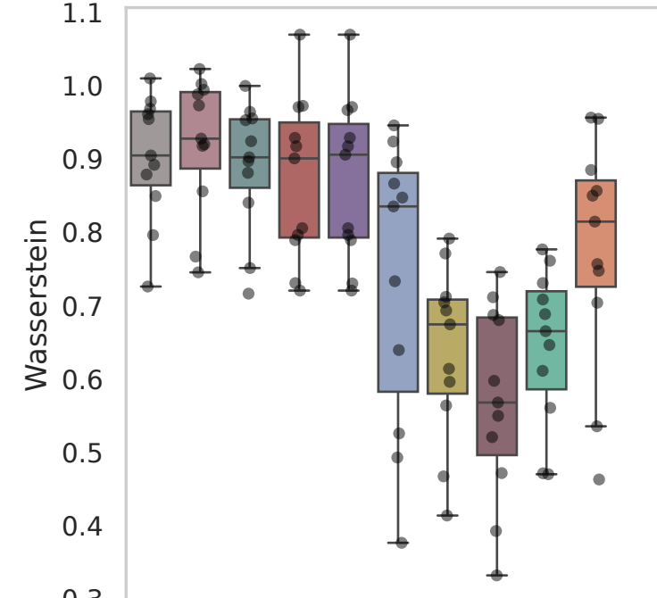
Dataset: Weinreb
