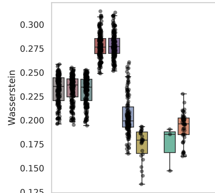
Dataset: Parse
