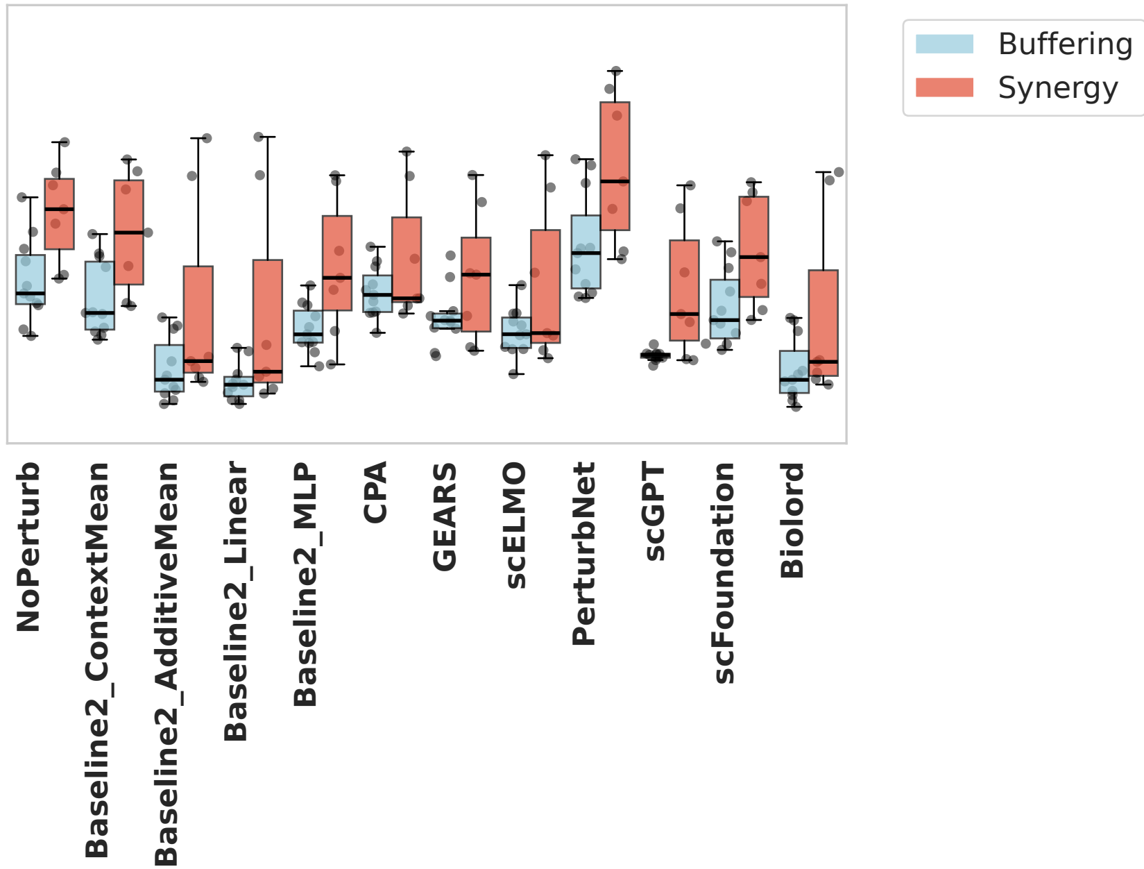
Seen2 Top20
