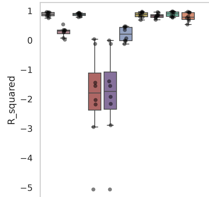
Dataset: Haber
