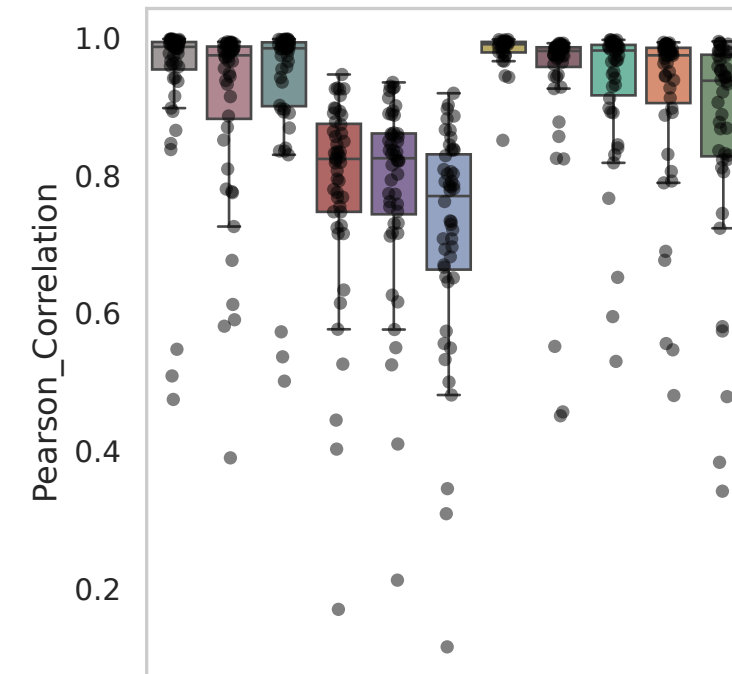
Dataset: Burkhardt
