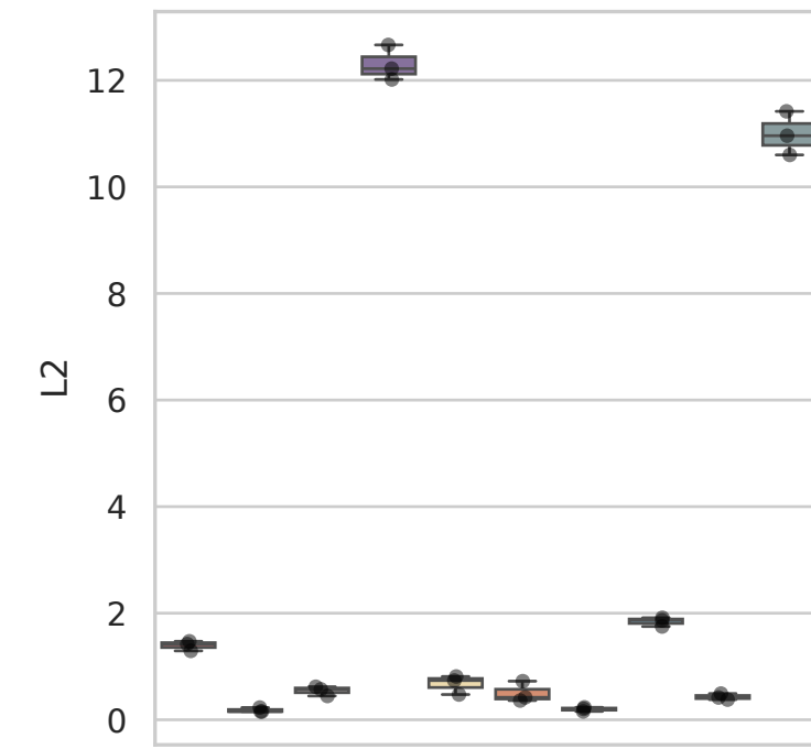
Dataset: Dixit
