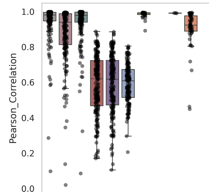
Dataset: Parse
