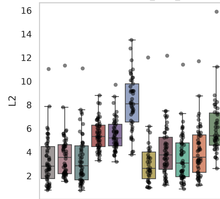
Dataset: Perturb_cmo_V1
