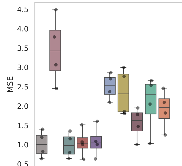
Dataset: Hagai
