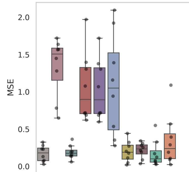
Dataset: Haber
