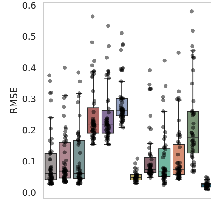
Dataset: Burkhardt
