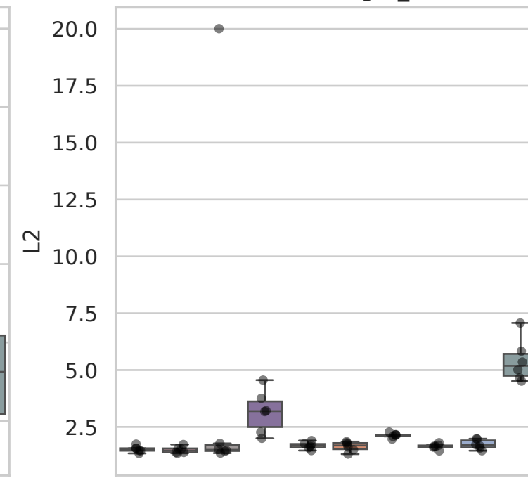
Dataset: Datlinger_2017
