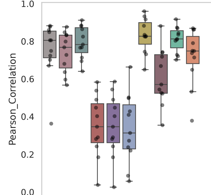
Dataset: Weinreb
