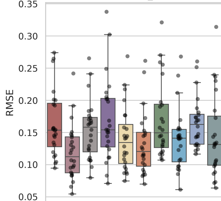
Dataset: Tian_crispra
