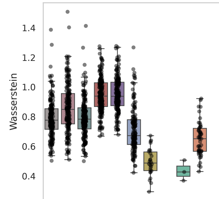
Dataset: Parse
