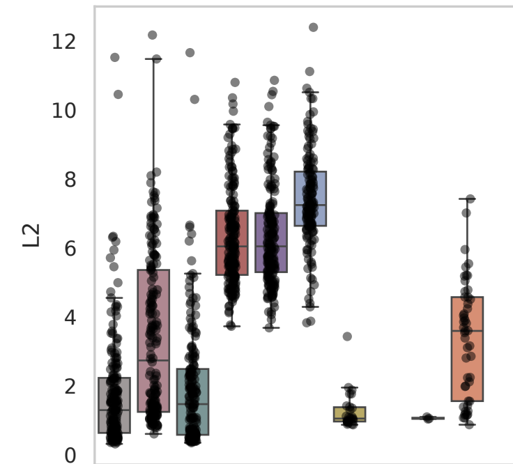
Dataset: Parse
