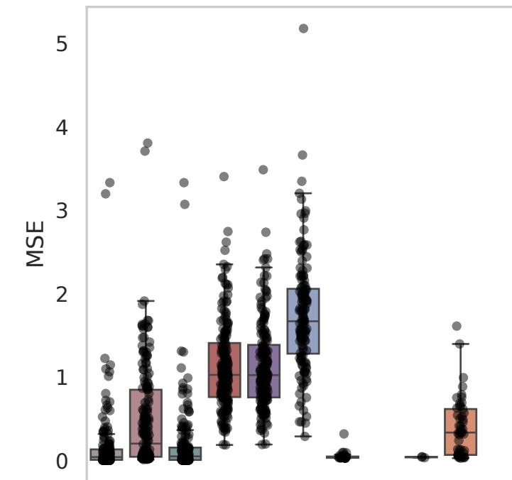
Dataset: Parse
