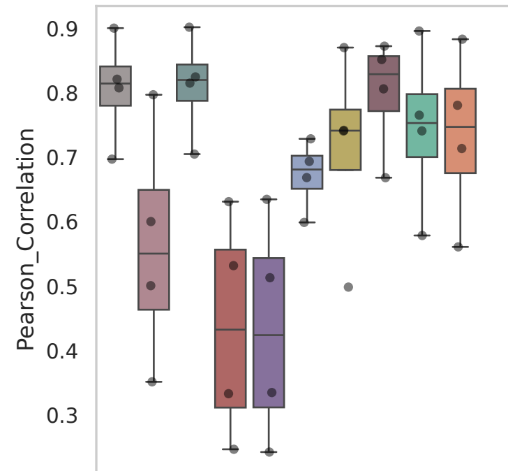
Dataset: Hagai
