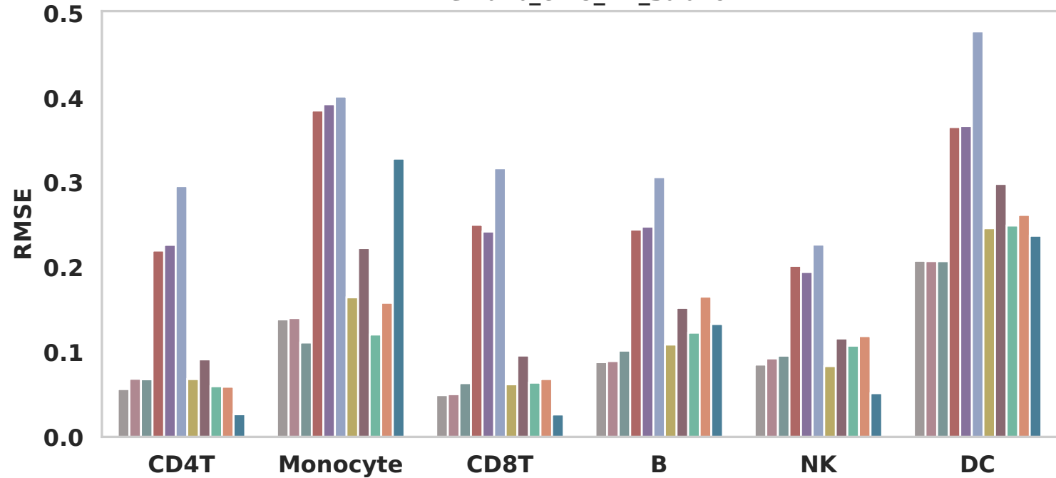
Perturb_cmo_V1_sub10
