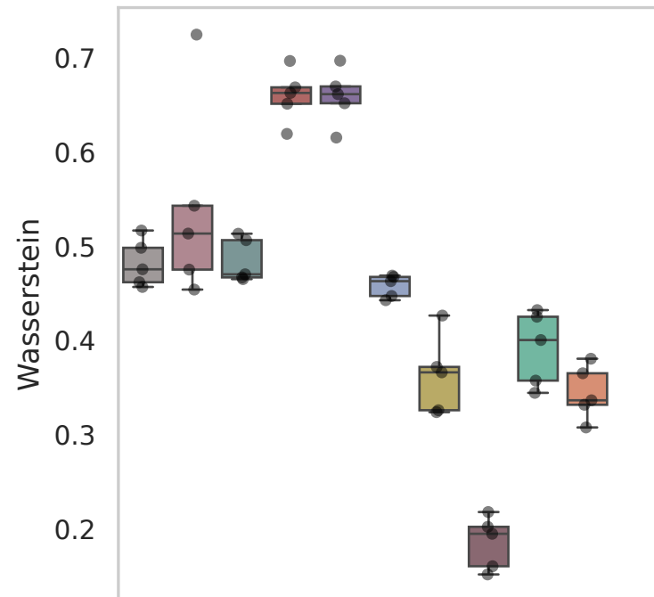
Dataset: Kang
