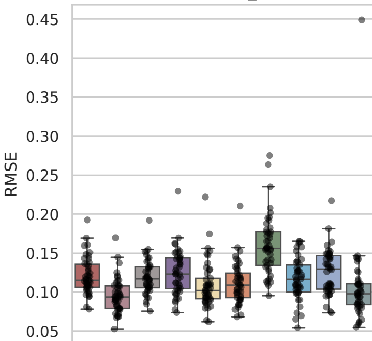
Dataset: Tian_crispri
