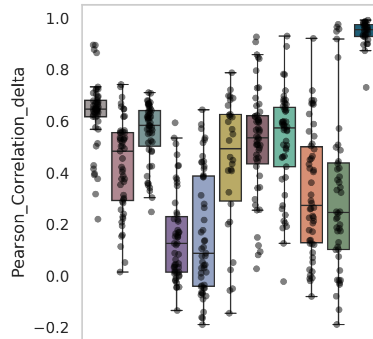
Dataset: Burkhardt
