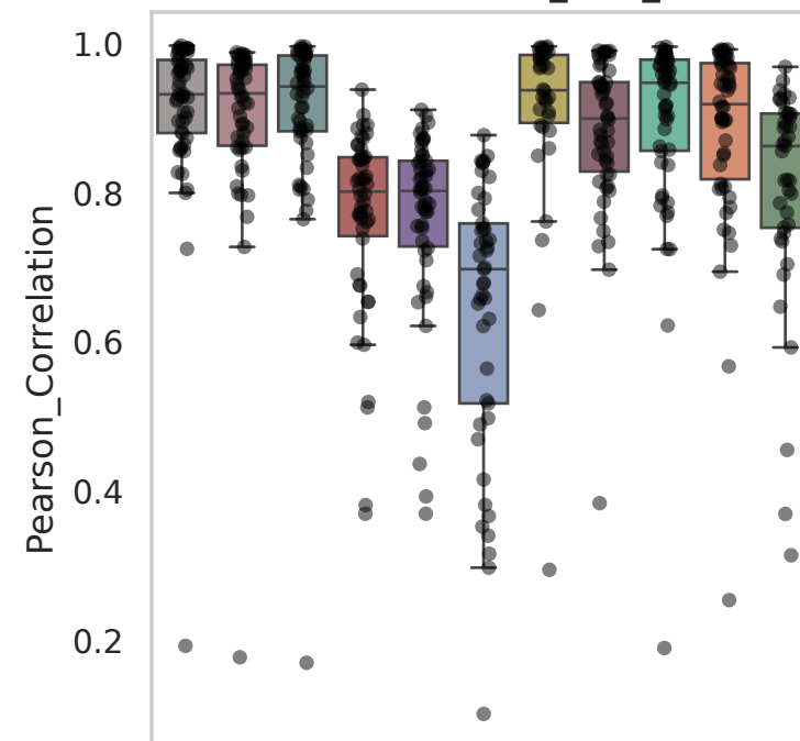
Dataset: Perturb_cmo_V1
