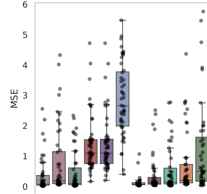
Dataset: Burkhardt
