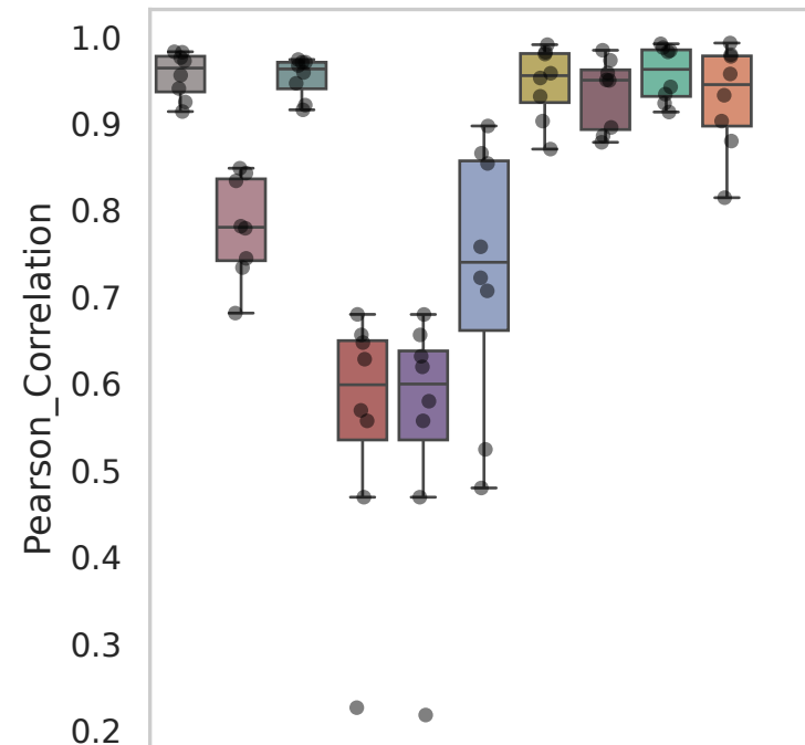
Dataset: Haber
