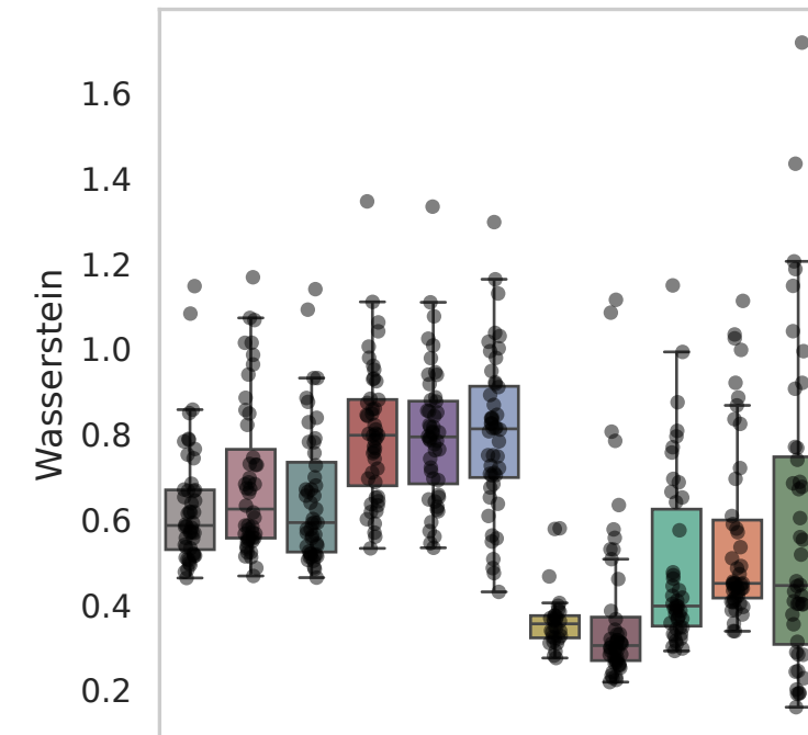
Dataset: Burkhardt
