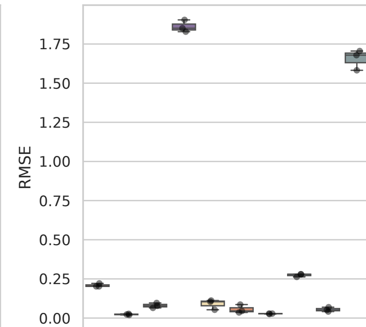
Dataset: Dixit
