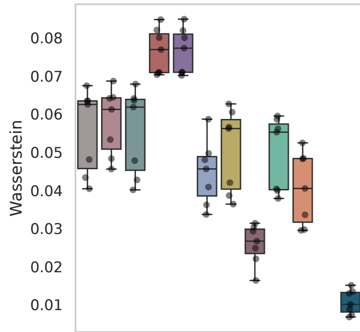
Dataset: Kang
