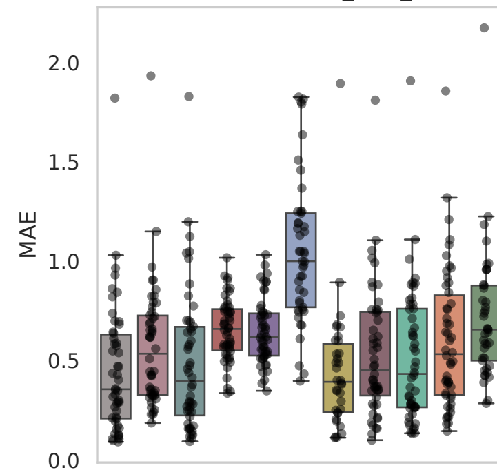
Dataset: Perturb_cmo_V1
