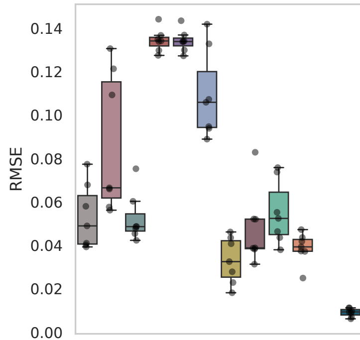
Dataset: Kang
