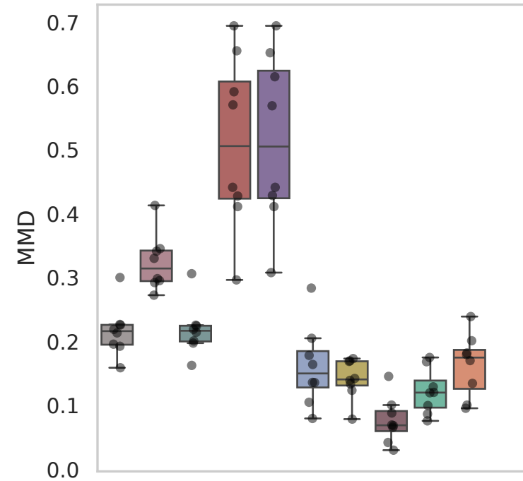
Dataset: Haber
