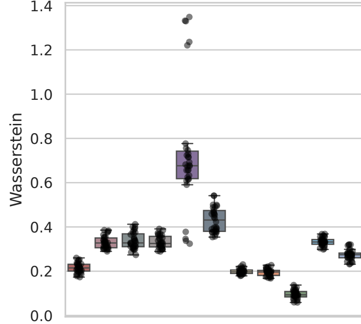
Dataset: Dixit
