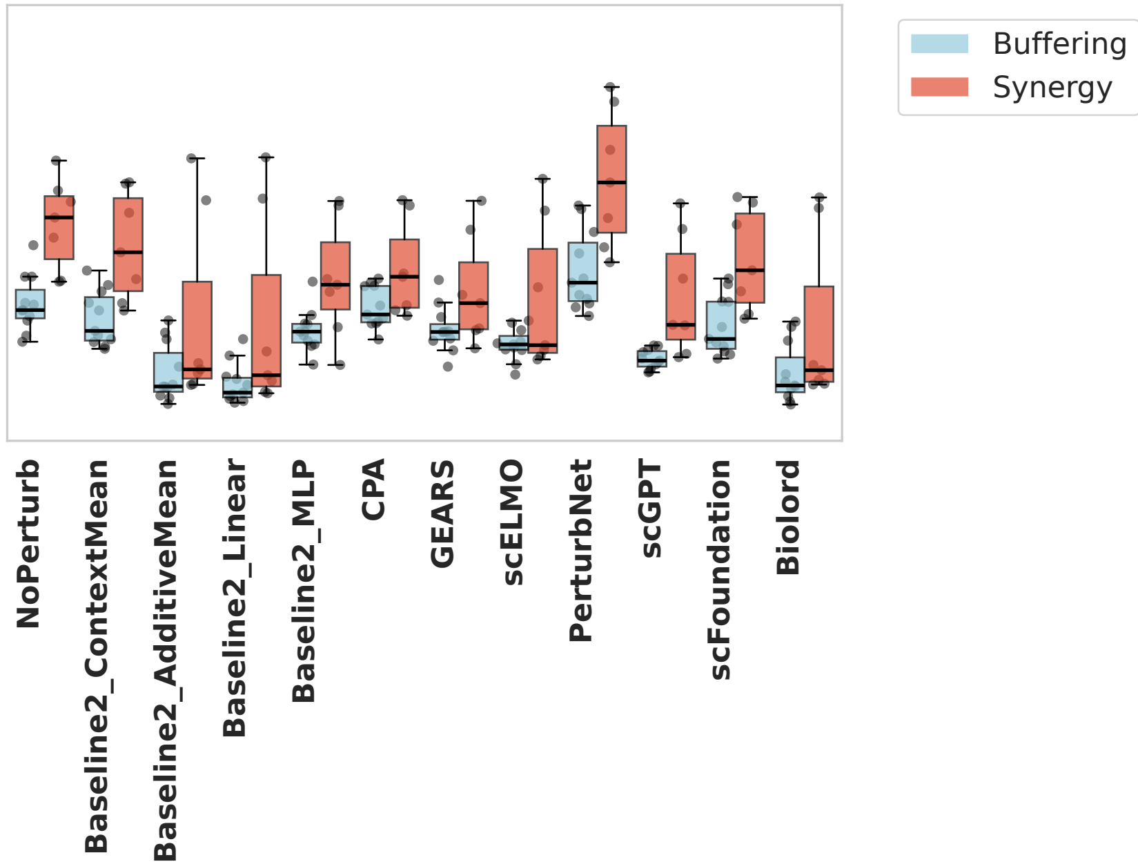
Seen2 Top50
