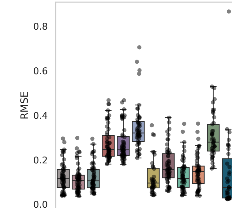
Dataset: Perturb_cmo_V1
