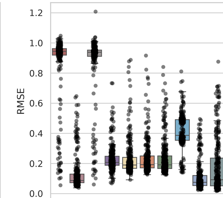
Dataset: Joung
