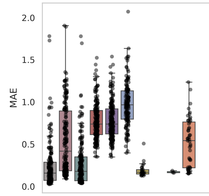
Dataset: Parse
