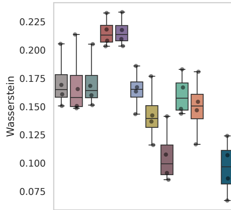
Dataset: Hagai
