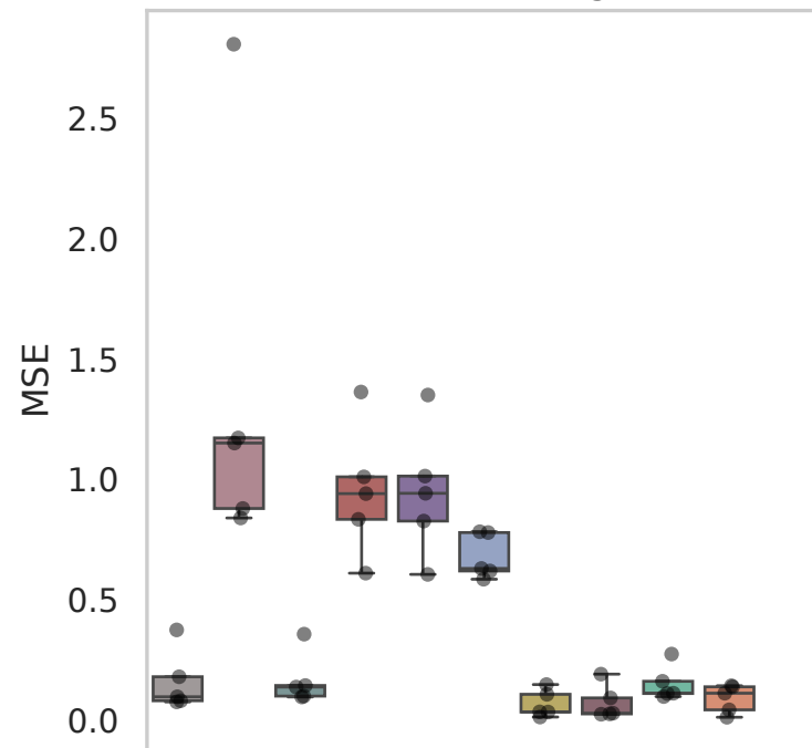
Dataset: Kang
