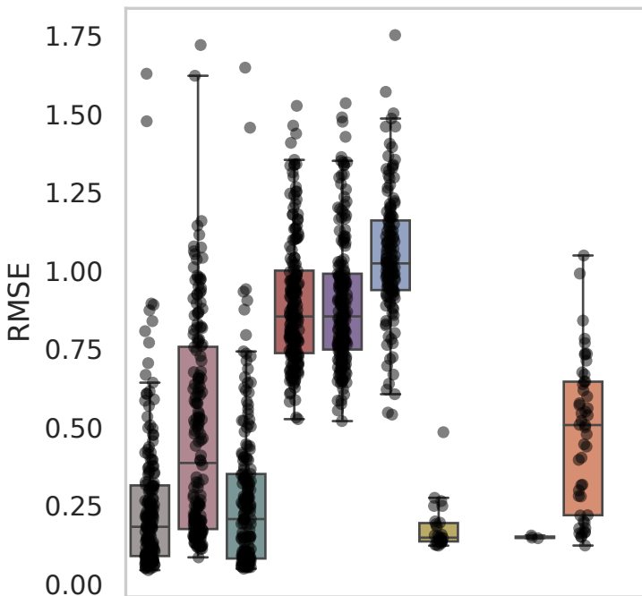
Dataset: Parse
