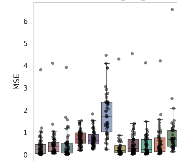
Dataset: Perturb_cmo_V1
