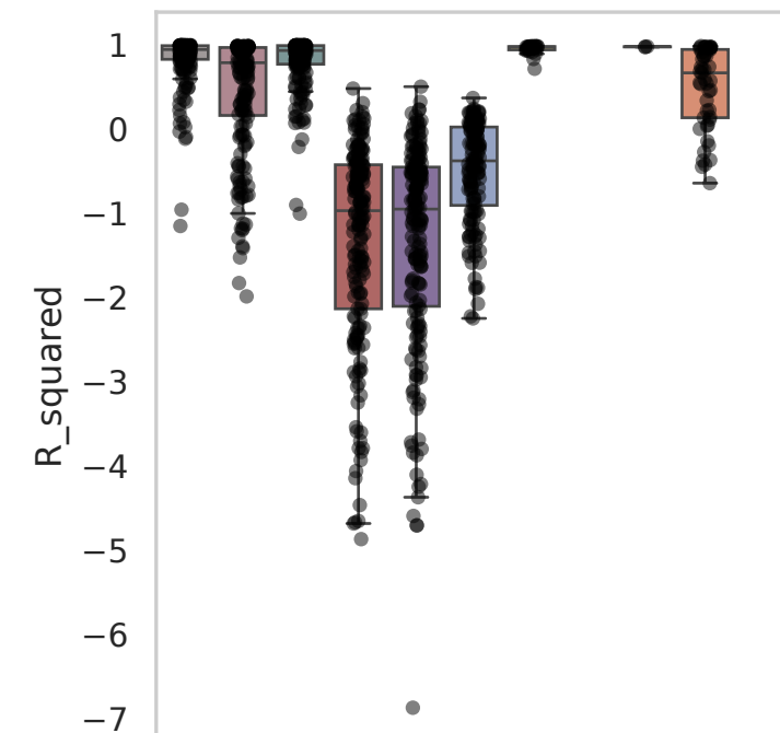
Dataset: Parse
