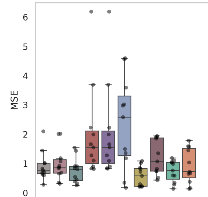
Dataset: Weinreb
