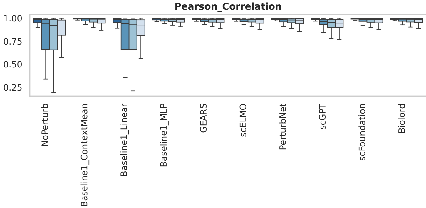
Pearson_Correlation
