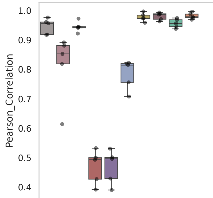
Dataset: Kang
