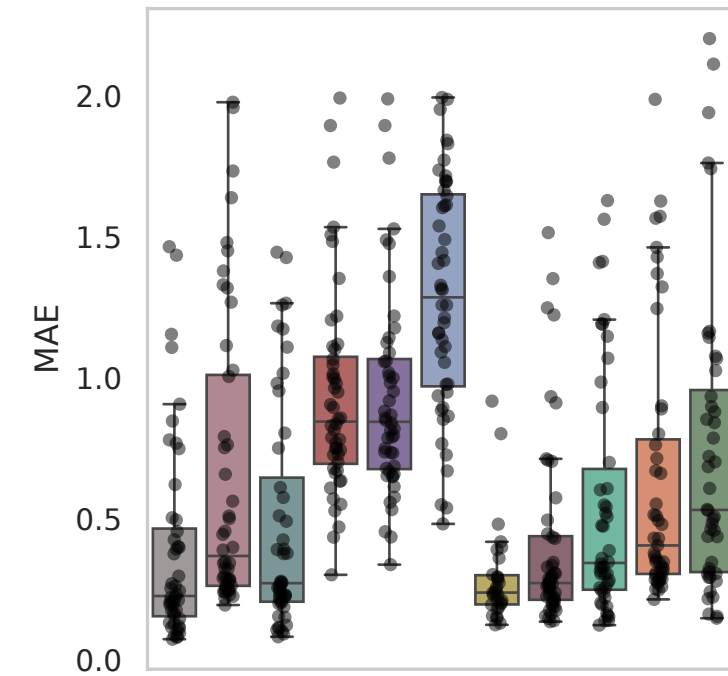
Dataset: Burkhardt
