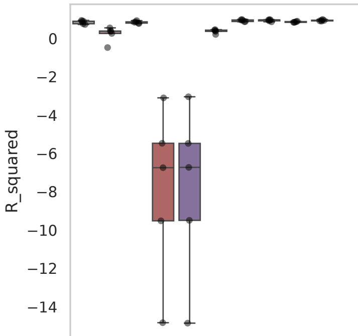
Dataset: Kang
