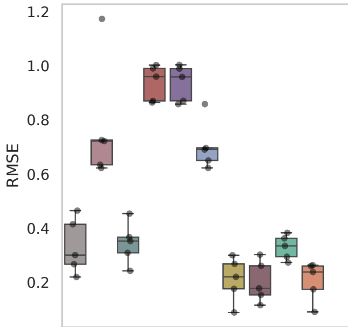
Dataset: Kang
