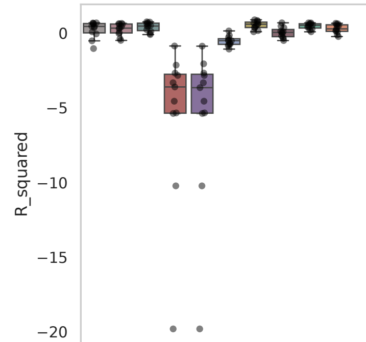
Dataset: Weinreb
