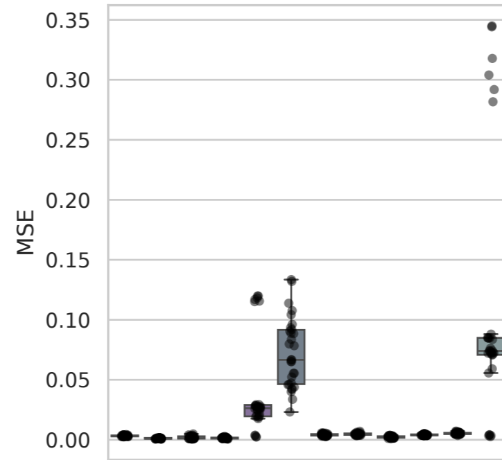
Dataset: Dixit
