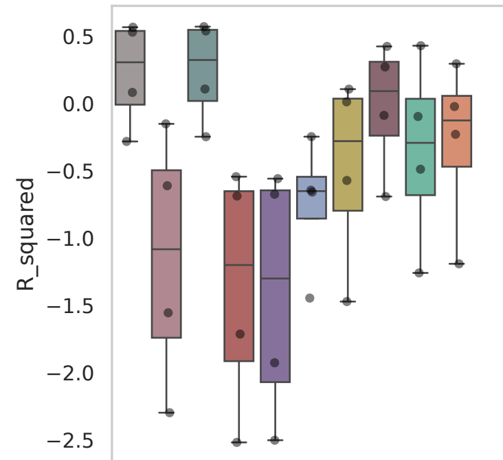
Dataset: Hagai
