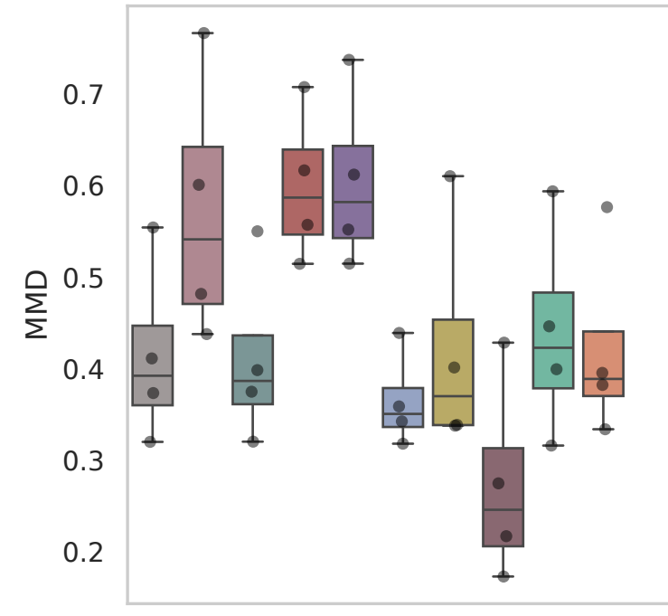
Dataset: Hagai
