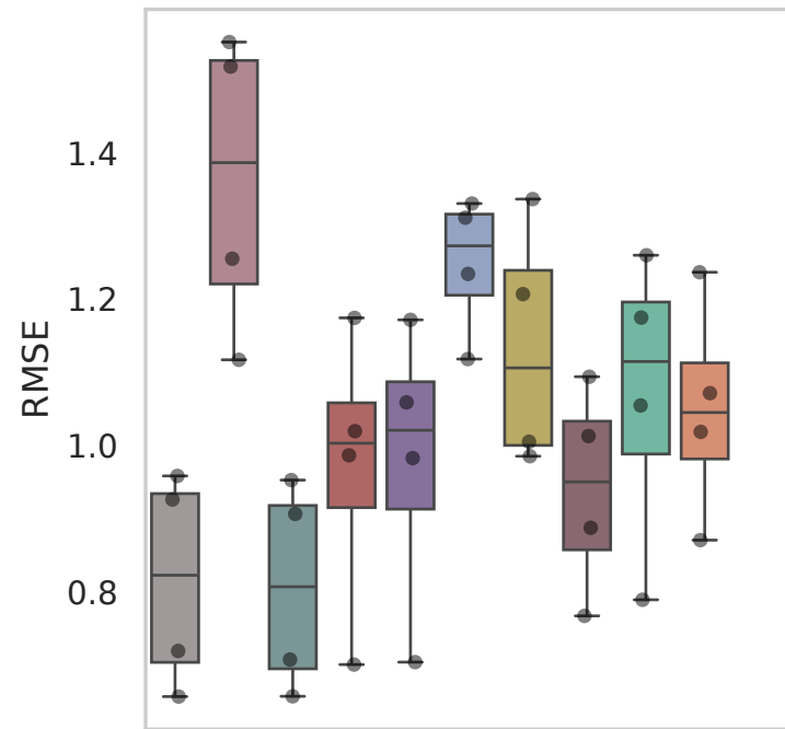
Dataset: Hagai
