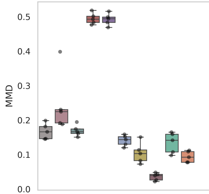
Dataset: Kang
