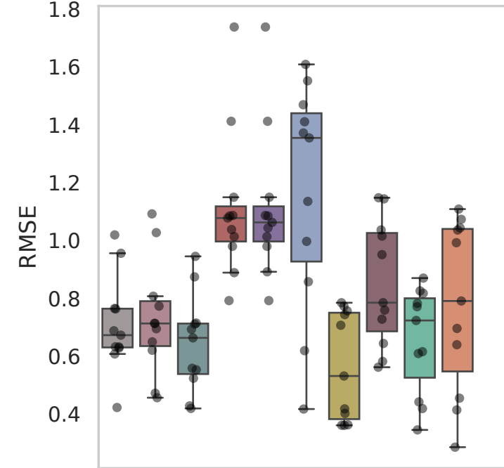
Dataset: Weinreb
