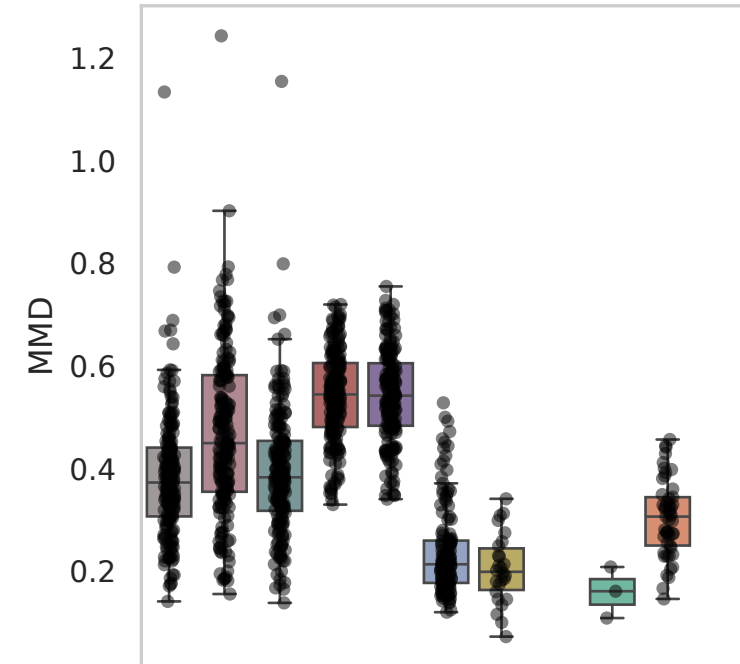
Dataset: Parse
