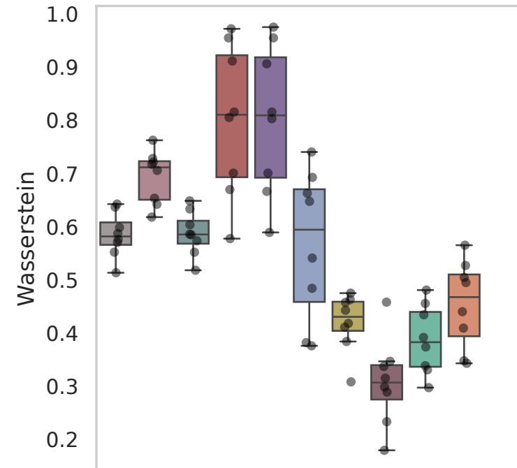
Dataset: Haber
