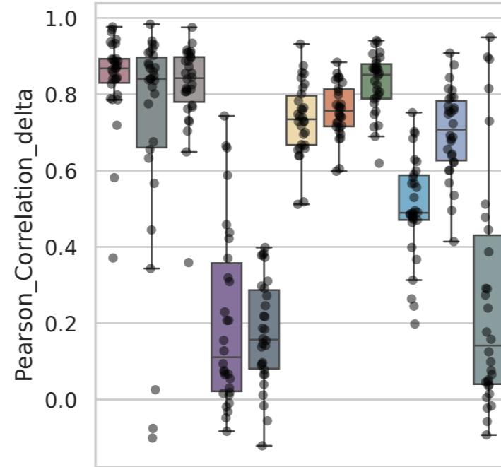
Dataset: Dixit
