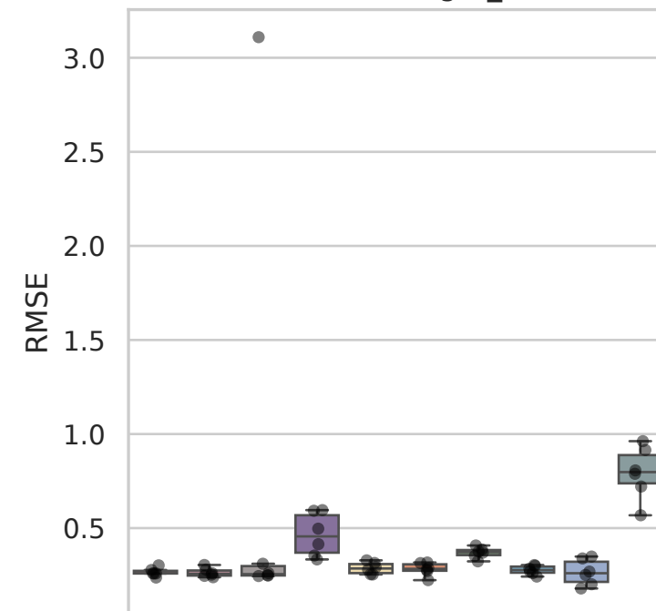
Dataset: Datlinger_2017
