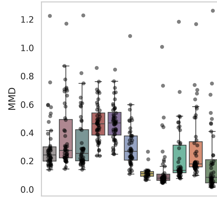
Dataset: Burkhardt
