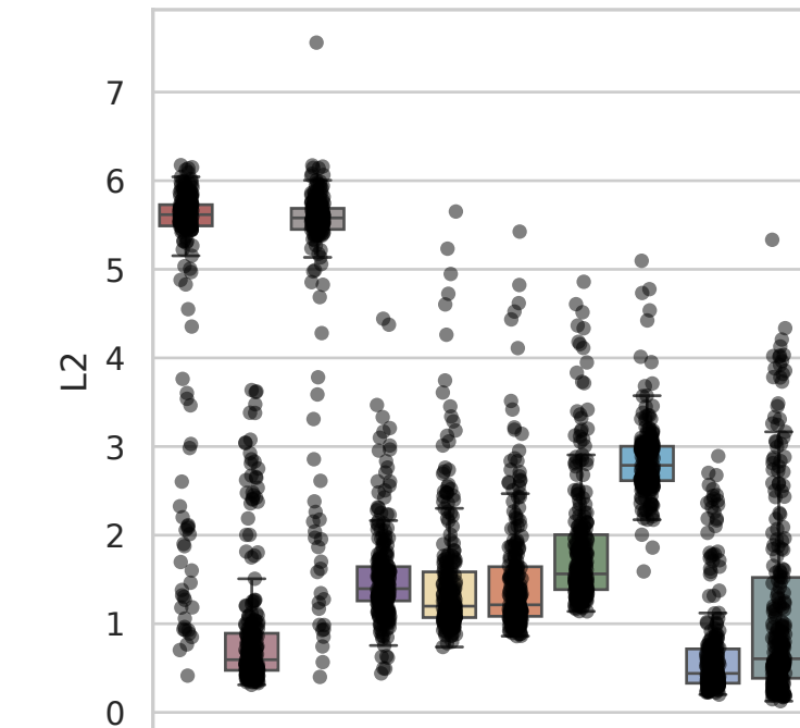
Dataset: Joungh
