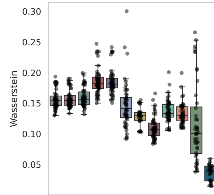
Dataset: Burkhardt
