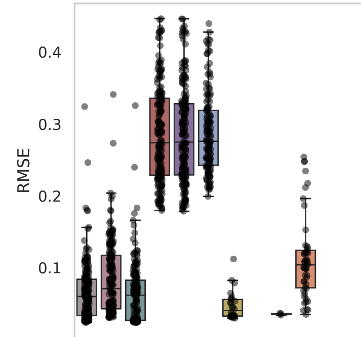
Dataset: Parse
