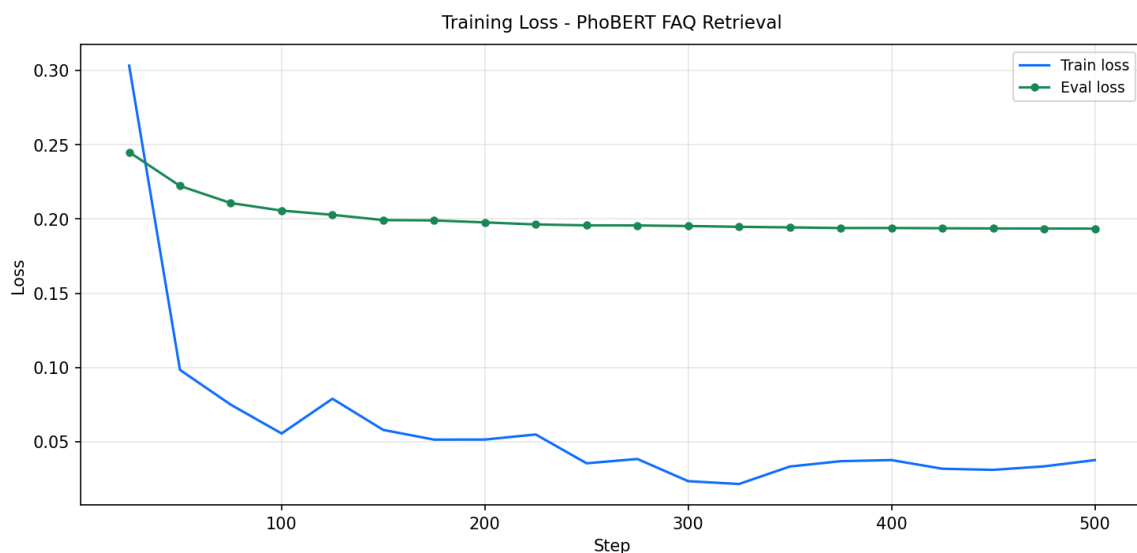
Hình 4.4: Đường cong loss trong quá trình huấn luyện PhoBERT Fine-tuned
