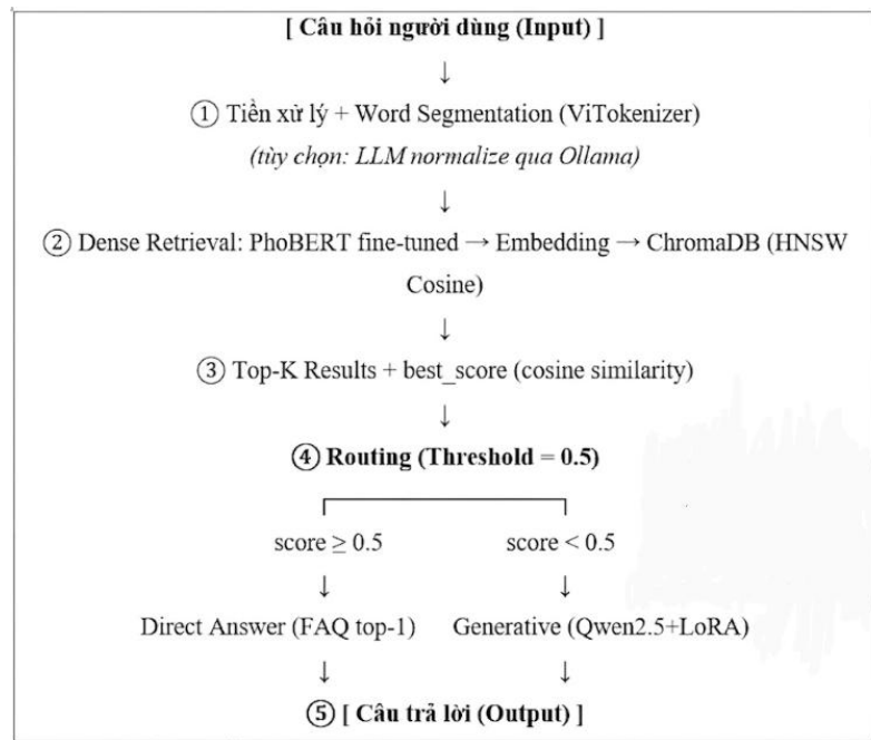
Hình 3.3: Kiến trúc tổng quan hệ thống Hybrid FAQ + Generative RAG (ngưỡng THRESHOLD trong cài đặt thực tế là 0.6)
