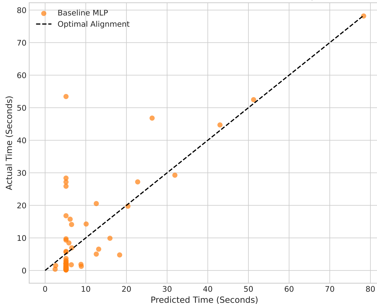
Baseline MLP: Predicted vs. Actual Latency
