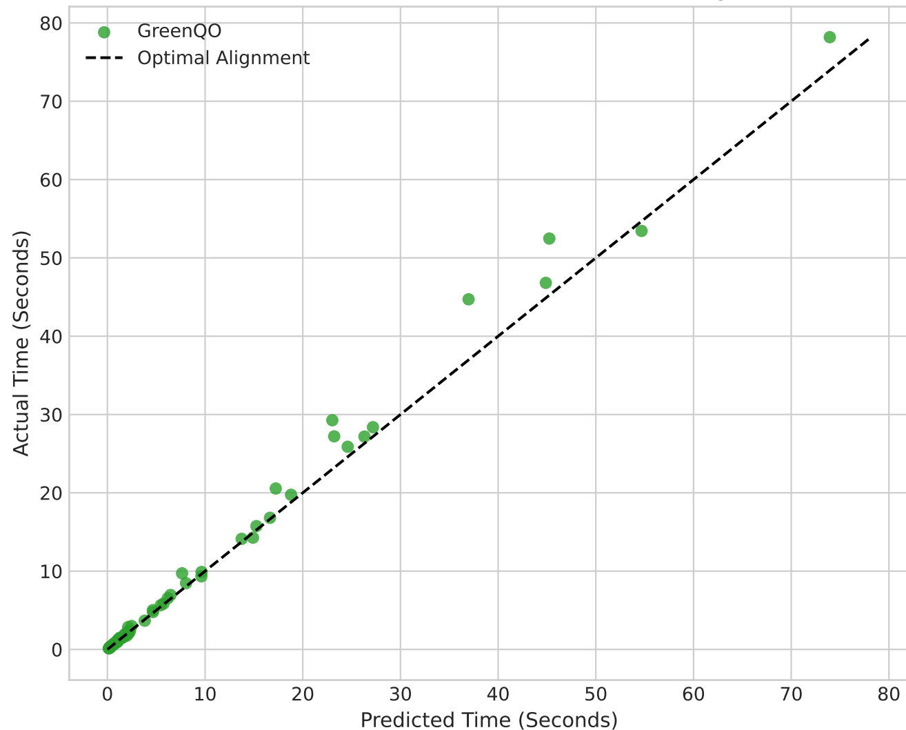
GreenQO: Predicted vs. Actual Latency
