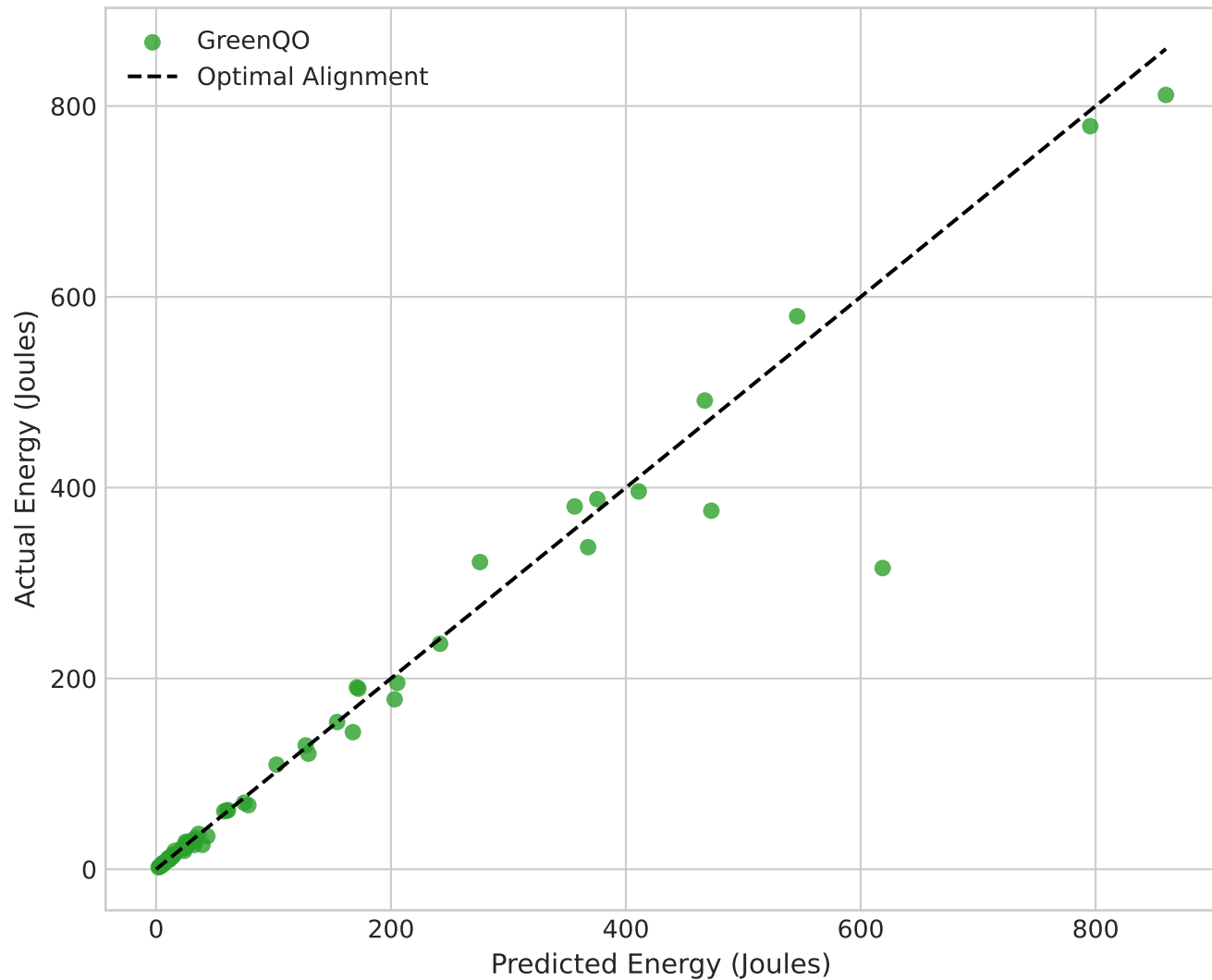
GreenQO: Predicted vs. Actual Energy
