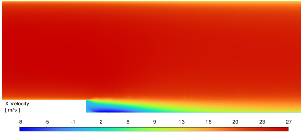
(B) SA contour for u_x .
