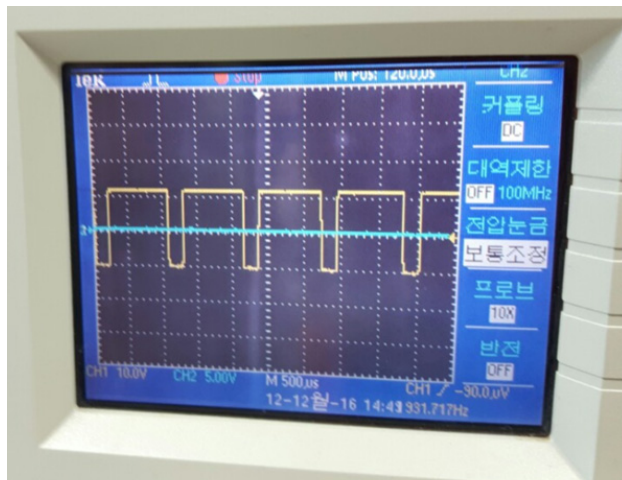
[그림 3-20] 오실로스코프 트리거 측정하기
