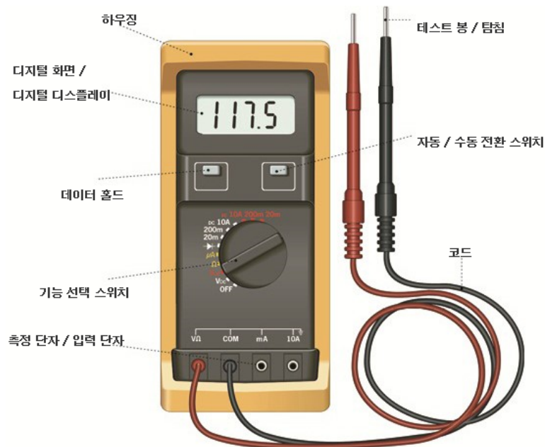
[그림 3-15] 디지털 멀티미터 상세 설명
