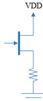
[그림 3-35] 출력 신호 - Pull Down
