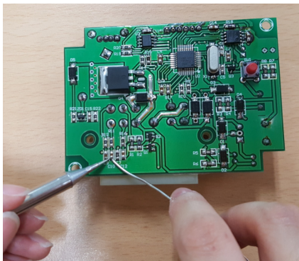
[그림 1-29] 인두기를 이용한 납땜 예시
