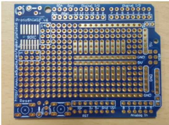
[그림 1-26] PCB 샘플 예시
