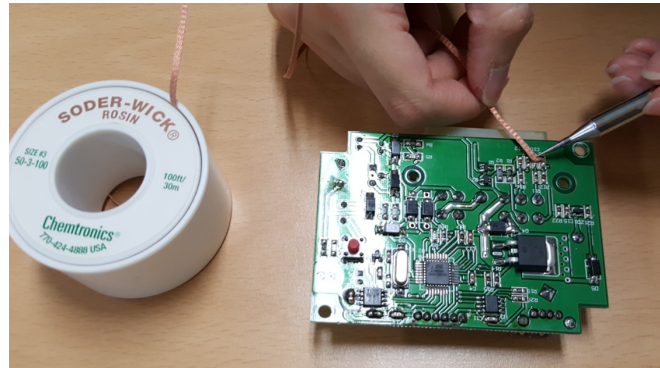
[그림 1-30] 솔더위크를 이용한 납 제거 예시
