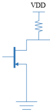
[그림 3-34] 출력 신호 - Pull Up
