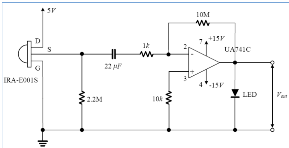
[그림 1-24] 초전형 적외선 센서를 이용한 인체 감지 실험용 회로도 예시
