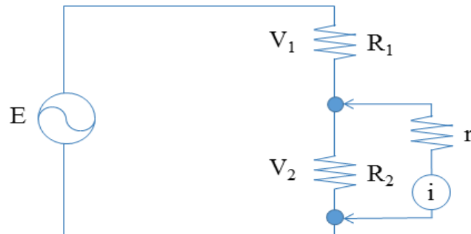
[그림 3-6] 전압 측정의 개념
