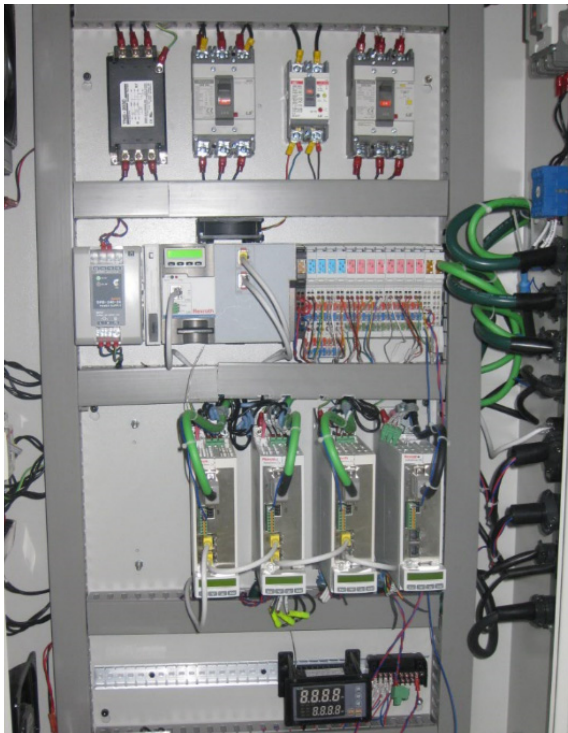
[그림 1-11] 범용로봇의 제어기 조작반
