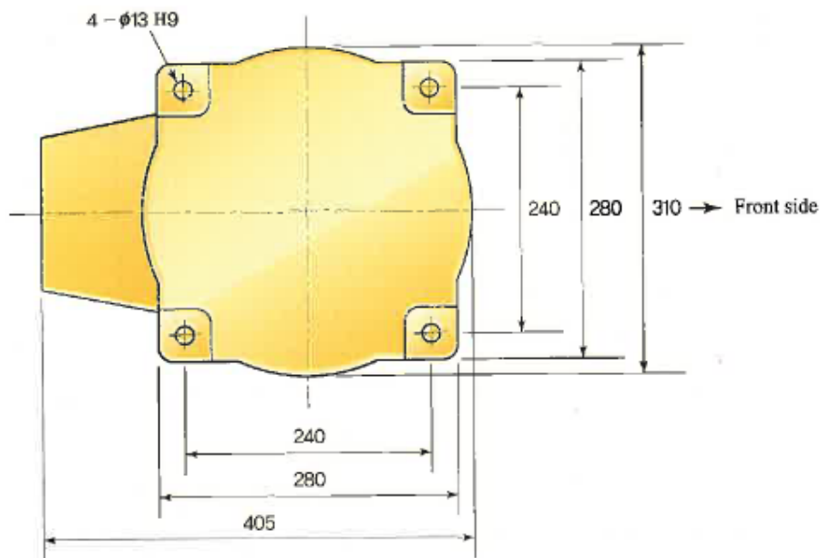
출처: OO전자(2015). 『OO로봇 RAS-2 사용자 매뉴얼』. OO로보틱스.. p.63 [그림 1-1] 로봇 지상 설치를 위한 기초 부분 사양 예
