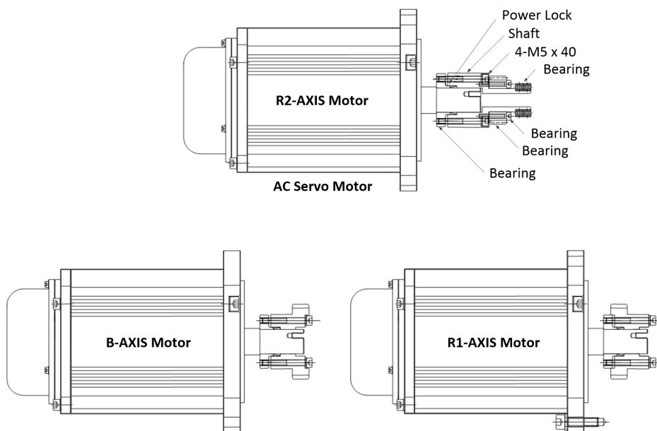
[그림 2-10] 손목축 모터 assembly
