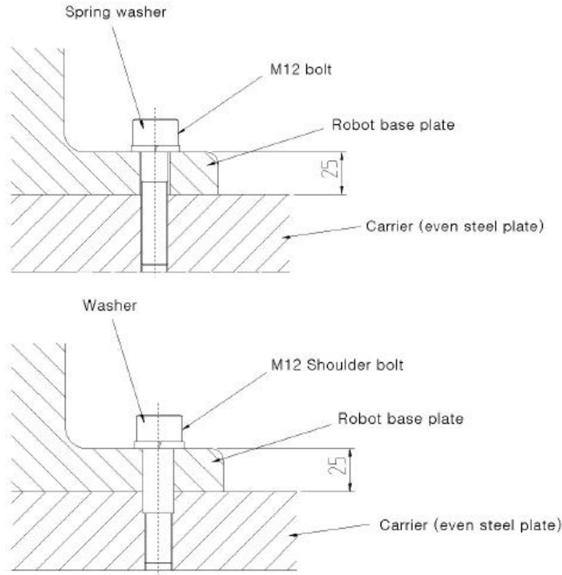
출처: OO전자(2015). 『OO로봇 RAS-2 사용자 매뉴얼』 . OO로보틱스.. p.65 [그림 1-4] 로봇 설치용 기초 플레이트
