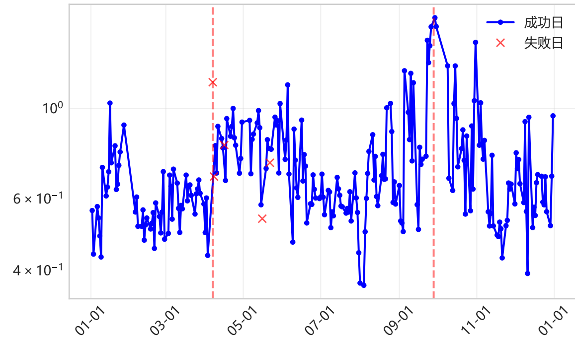
波动率的波动率 \sigma (对数坐标)
