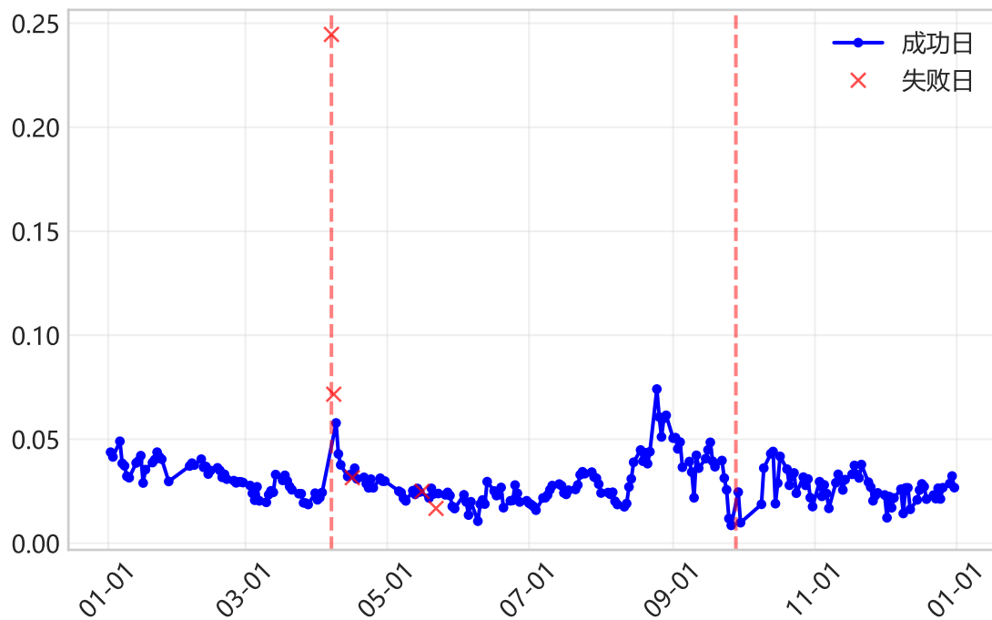
初始方差 v_0
