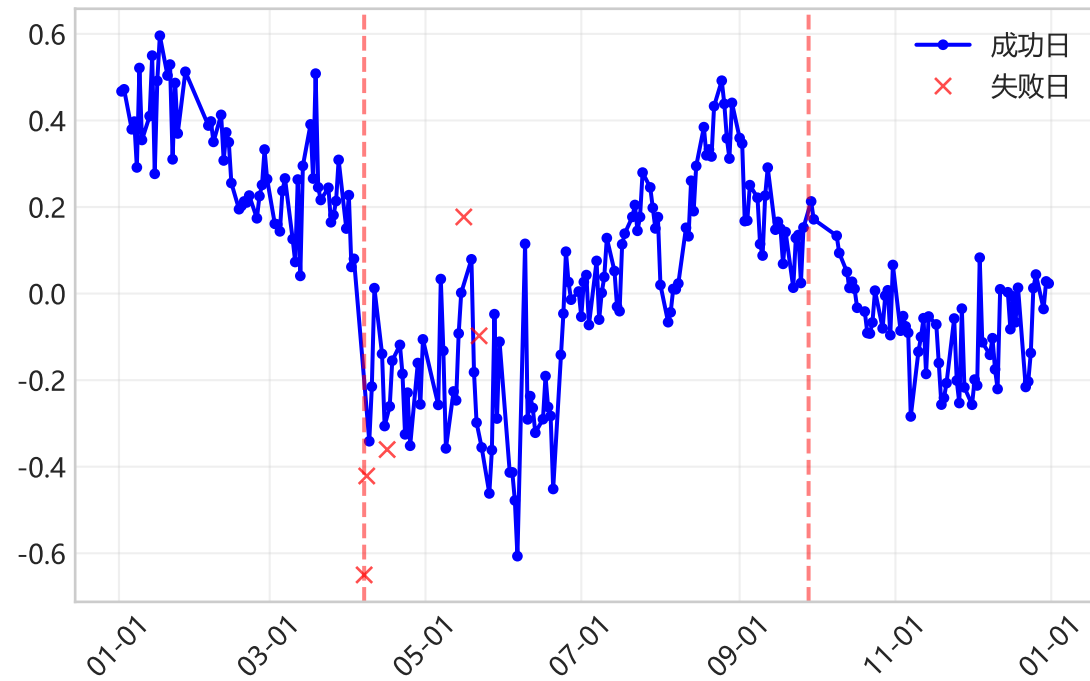
相关系数 \rho
