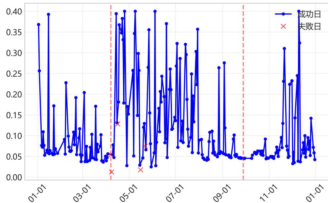
长期方差 \theta
