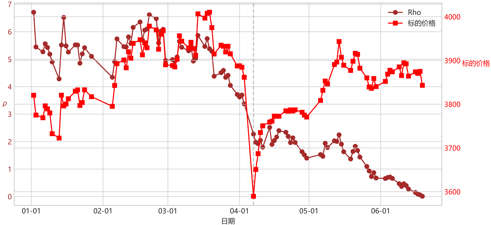
Rho 与标的价格动态
