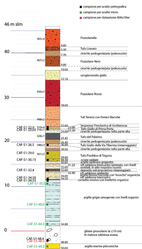
Fig. 5 - Stratigrafia del sondaggio S1 (from Parotto, 2026).
