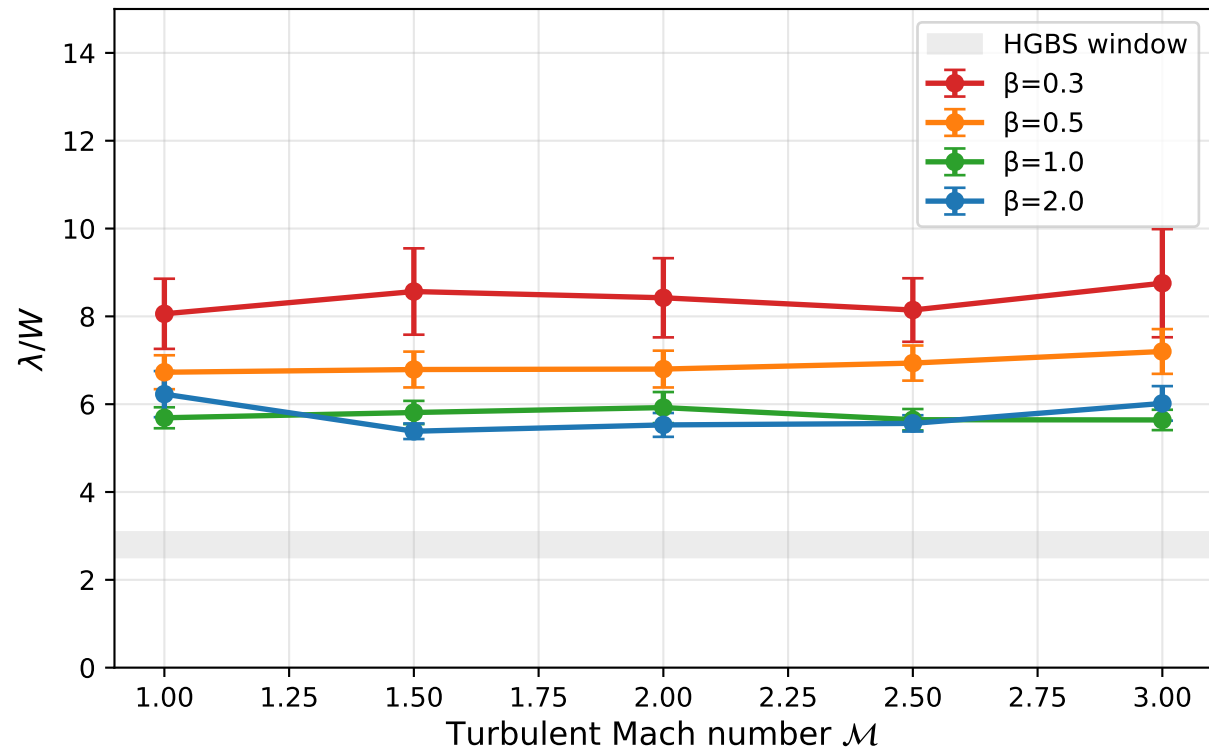
(a) Longitudinal field: \lambda/W vs \mathcal{M} per \beta (n=80 per cell, error = s.e.m.)
