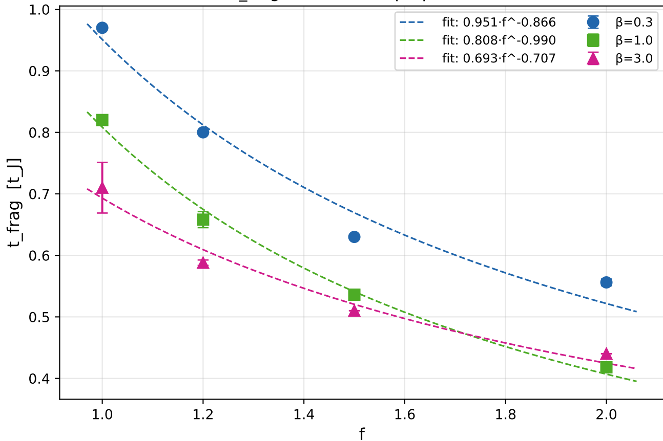
PFS: t_{\text{frag}} vs f ( \theta=90^\circ , perpendicular B)
