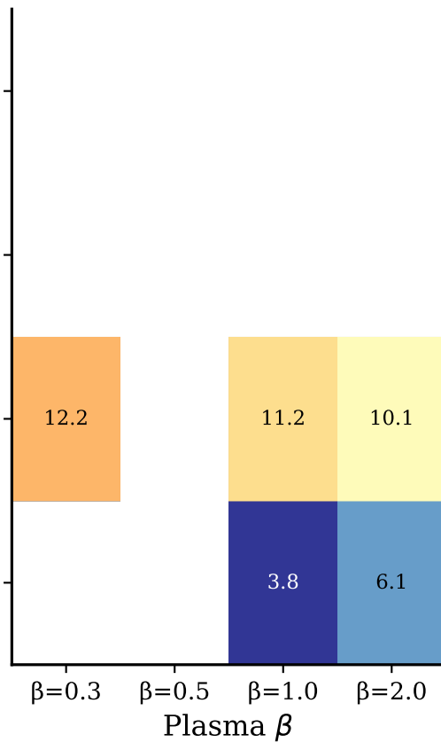
Solenoidal (NC)
