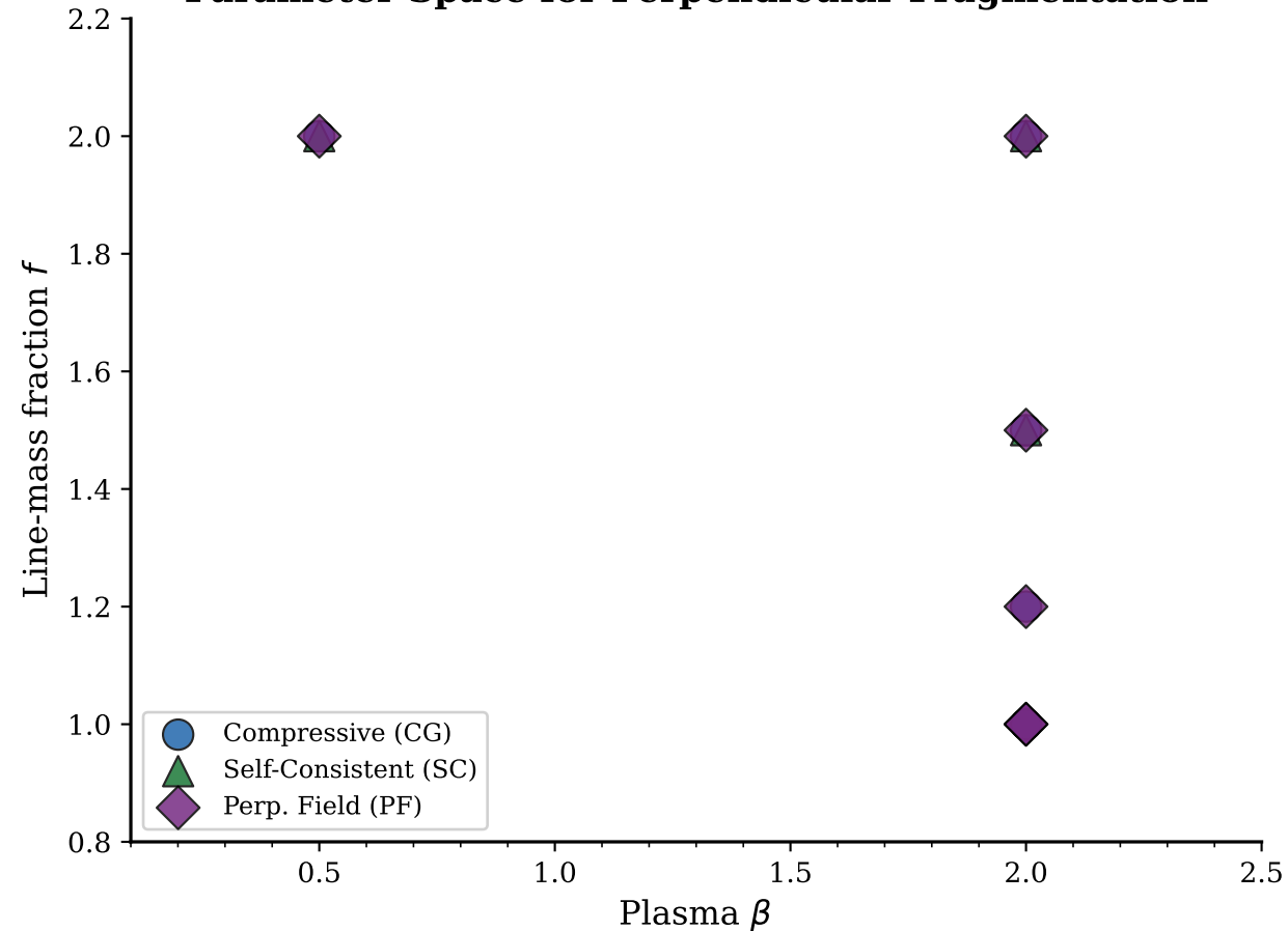
Parameter Space for Perpendicular Fragmentation
