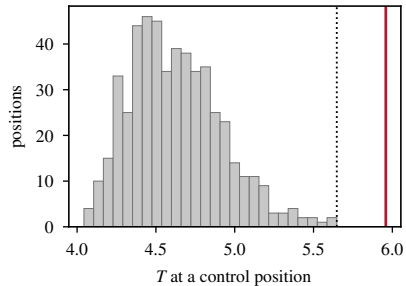
(d) the 512 controls
