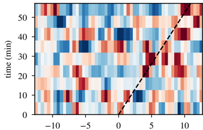
(d) the 512 controls
