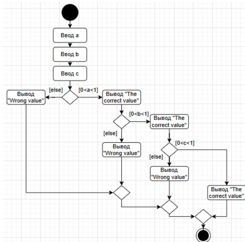
Рис. 16- UML-диаграмма к индивидуальному заданию 2.
