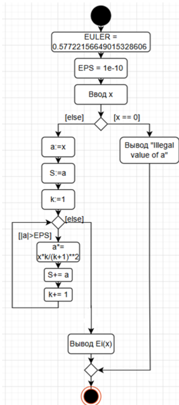
Рис. 10 – UML-диаграмма к примеру 5.
