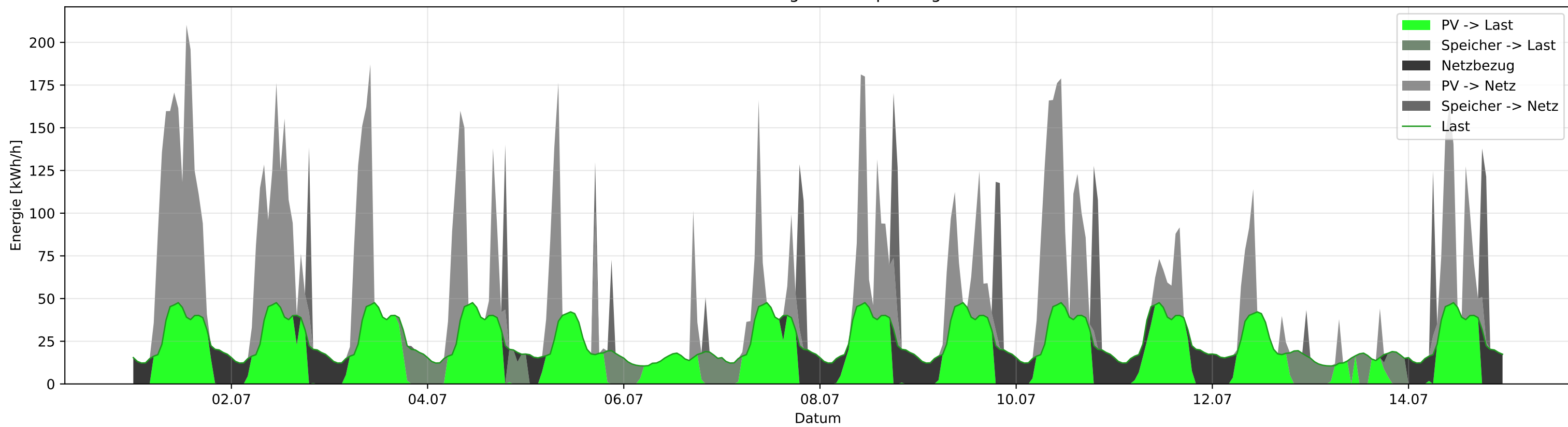
Lastdeckung und Einspeisung
