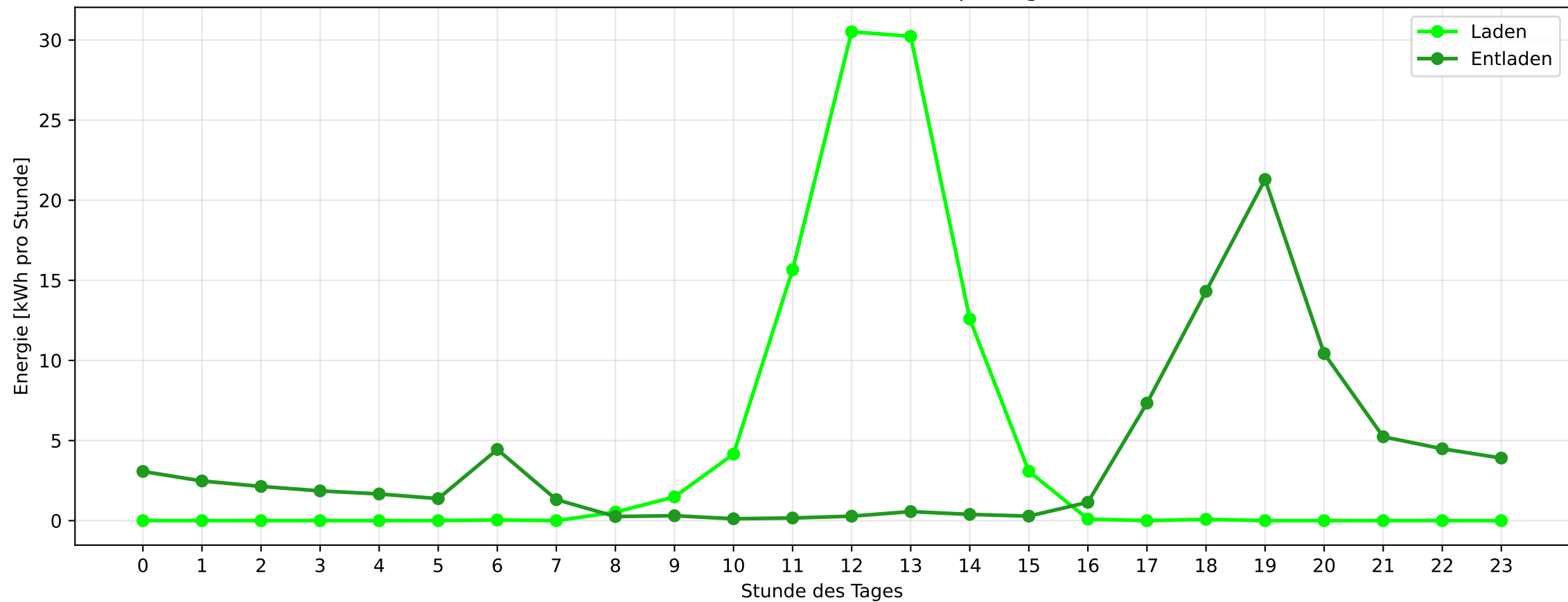
Gemittelte Lade-/Entladezeiten pro Tag
