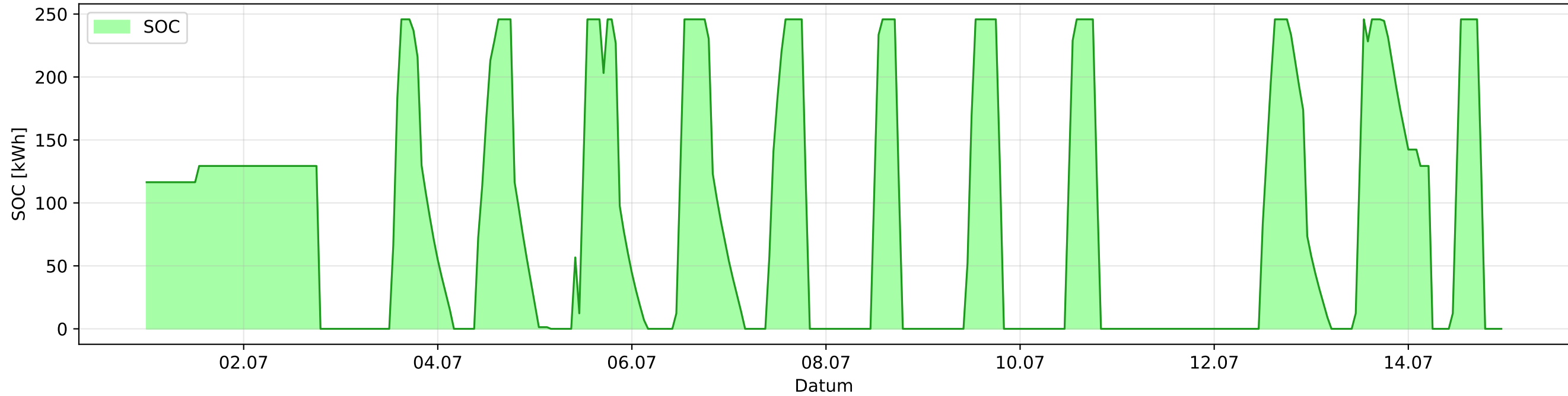
SOC über 14 Tage ab 2024-07-01
