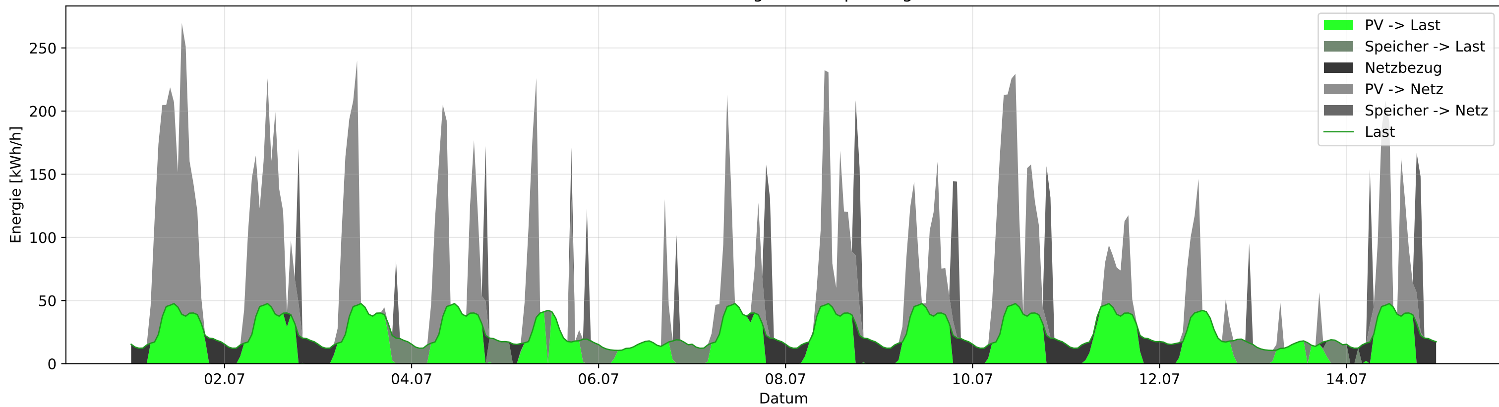
Lastdeckung und Einspeisung
