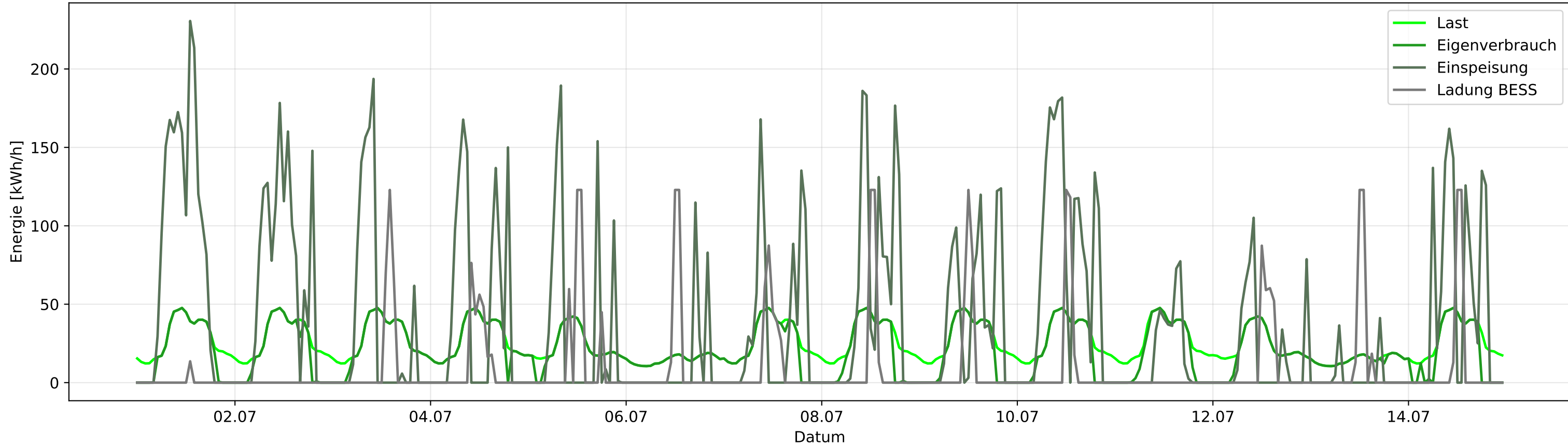
Last, Eigenverbrauch, Einspeisung und BESS-Ladung
