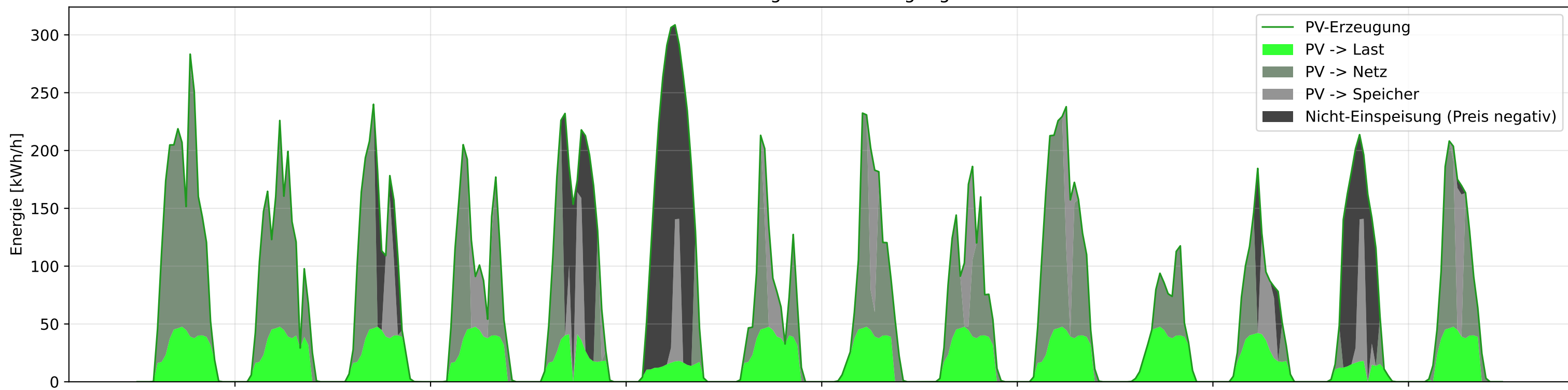
Lastdeckung und Einspeisung
