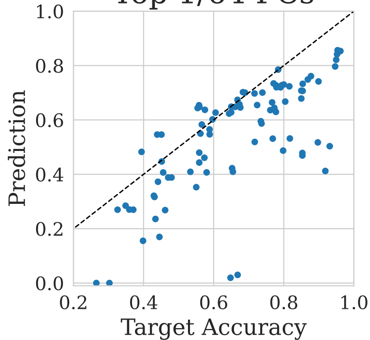
Top 1/64 PCs
