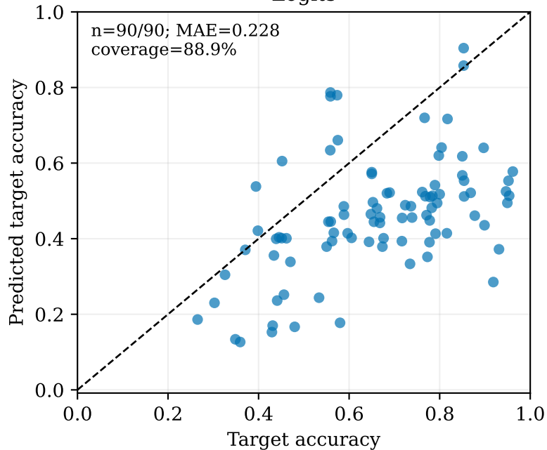
Logits
