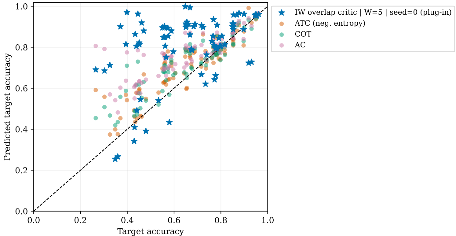
Logits
