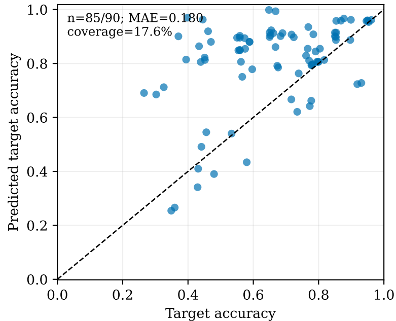
Logits
