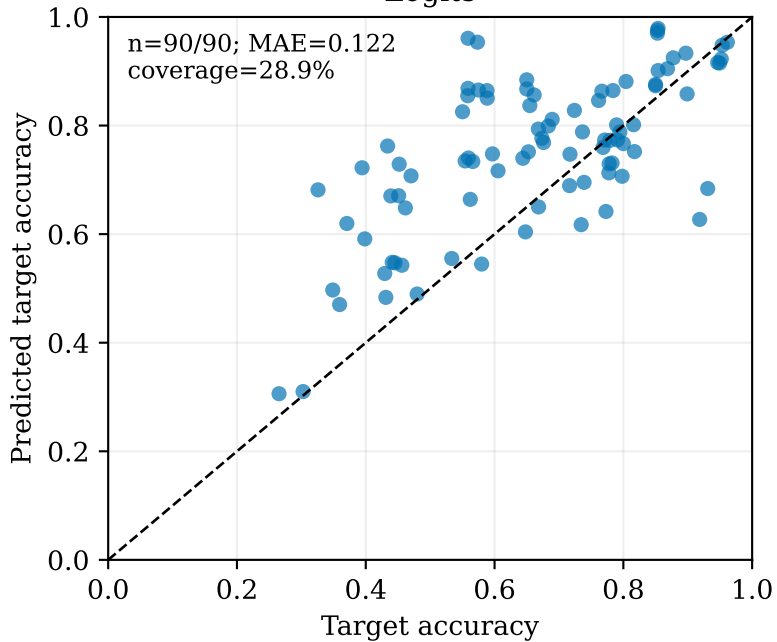
Logits
