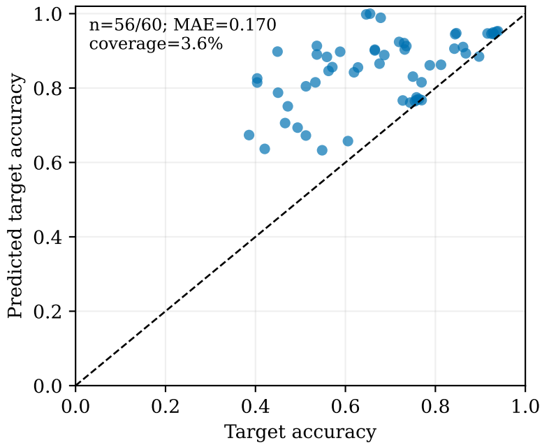
Logits
