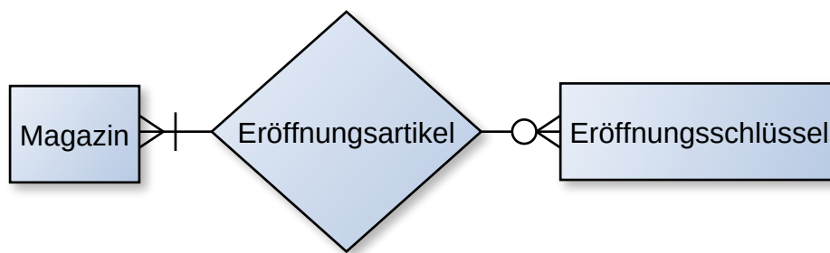
Abbildung 1: Entity-Relationship Diagramm des Datenmodells der Anwendung
