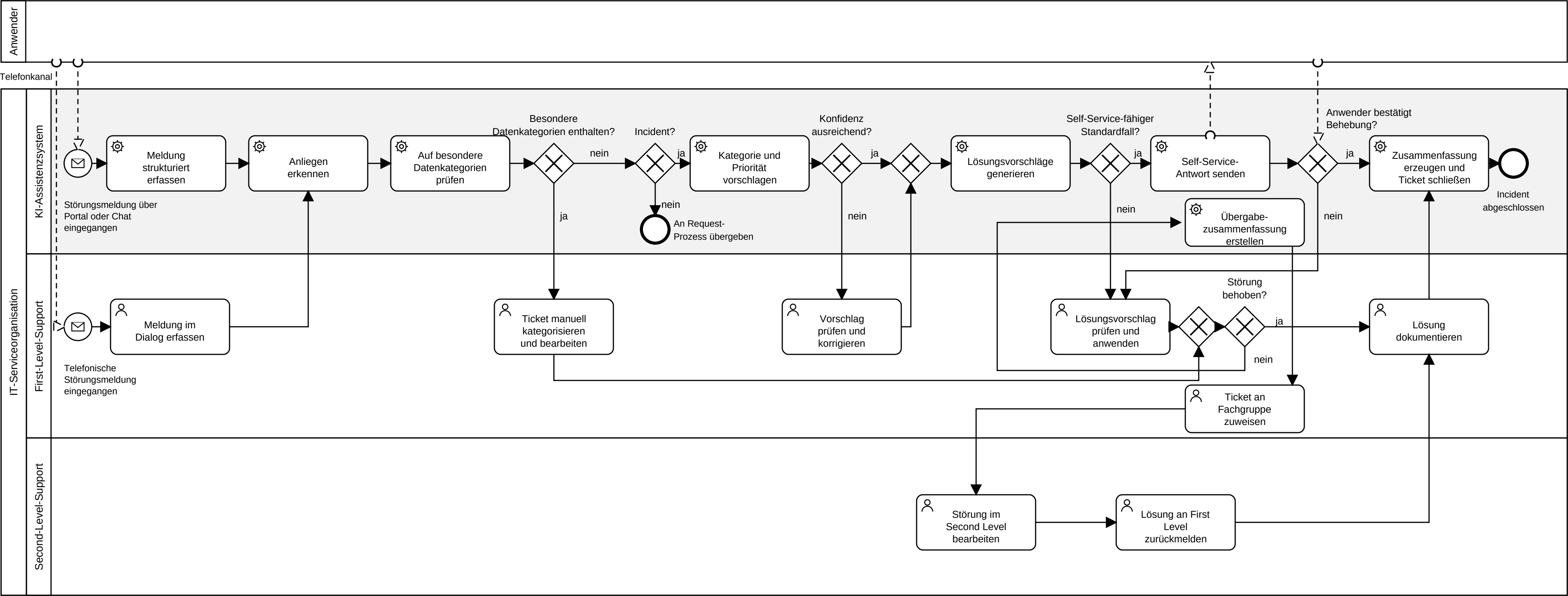
Zahnrad: maschinell ausgeführter Service Task – Person: menschlich ausgeführter User Task. Gestrichelt: Nachrichtenflüsse zwischen Anwender und IT-Serviceorganisation. Zwei Nachrichten-Startereignisse: Portal/Chat in der KI-Lane, Telefon in der First-Level-Lane.
