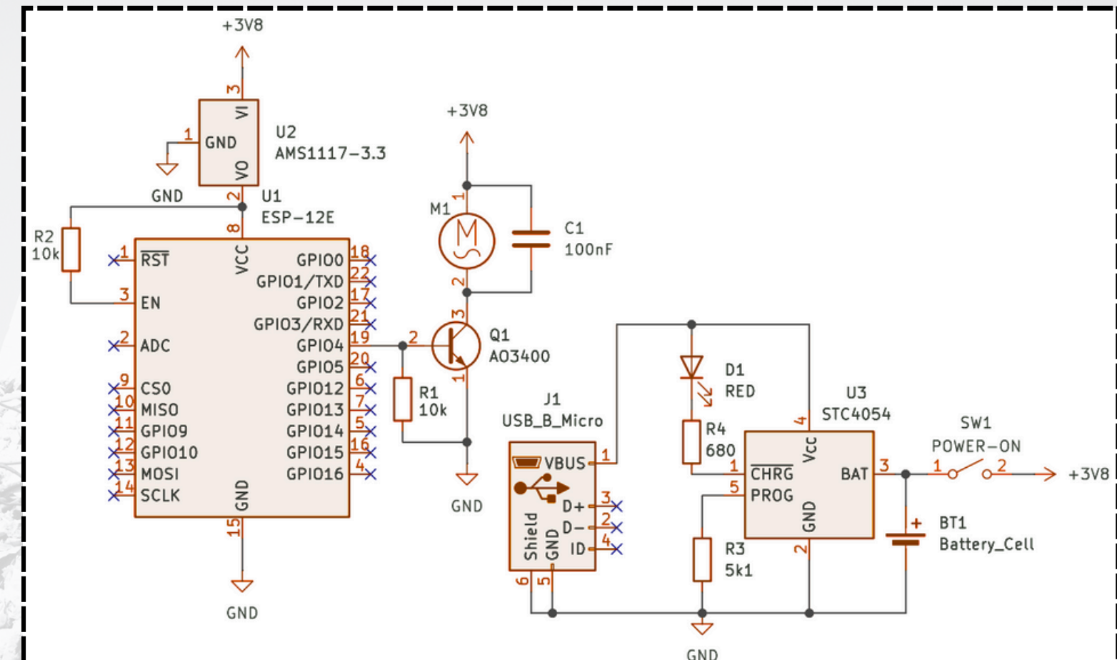
ПРИНЦИПИАЛЬНАЯ СХЕМА
