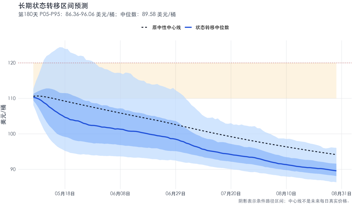
图 30 R/ggplot2 长期状态转移区间预测。双层阴影分别表示 5%–95% 和 25%–75% 条件区间，虚线为原中性中心路径。
