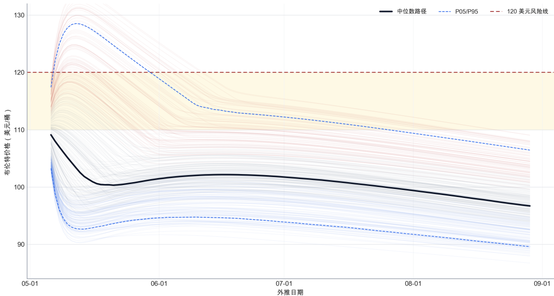
图 28 传统蒙特卡洛路径云图。图中从 2000 条模拟路径中分层抽取代表路径，黑线为中位数路径，蓝色虚线为 P05/P95 条件边界，红色虚线为 120 美元/桶风险线。
