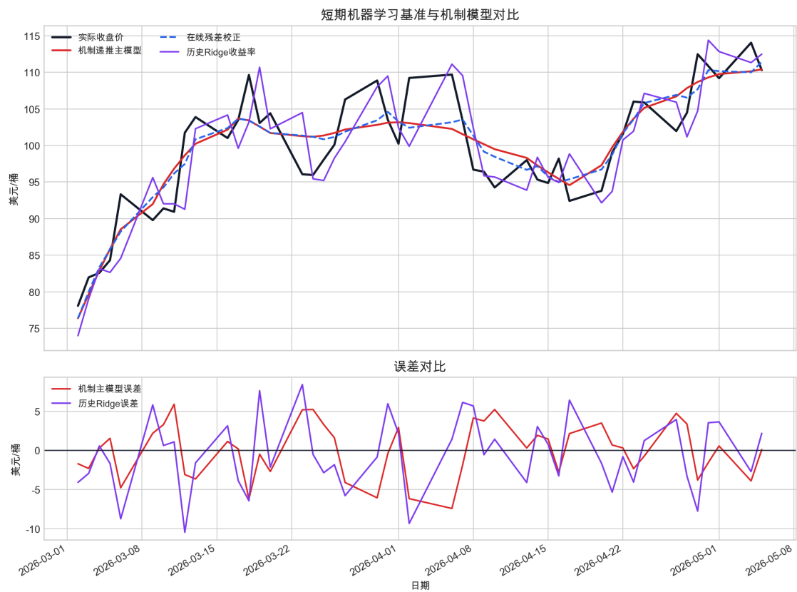
图 15 短期机器学习辅助层对比。Ridge 使用冲突前历史滞后价格特征训练，只作为机制路径的低自由度收益率修正。
