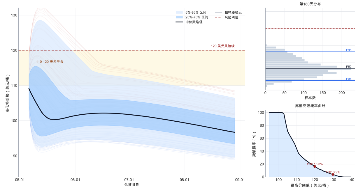
图 22 长期情景预测主图：蒙特卡洛情景树高级组合图。左侧展示中心路径、抽样路径云和 5%–95% / 25%–75% 条件区间，右上展示第 180 天终点分布，右下展示外推期突破 120、130 美元/桶的累计概率曲线。
