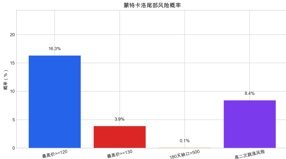
图 29 蒙特卡洛尾部风险概率。
