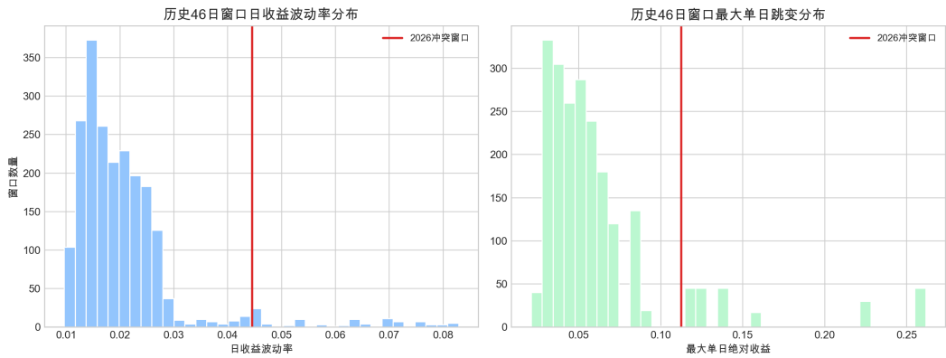
图 27 历史波动参数校准。2017–2025 同长度窗口为长期蒙特卡洛和状态转移扰动提供历史尺度。
