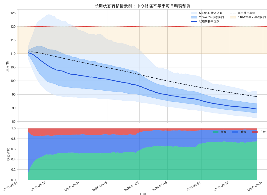
图 24 长期状态转移情景树。上图为状态转移后的价格扇形区间，下图为缓和、维持、升级三类状态的样本占比。
