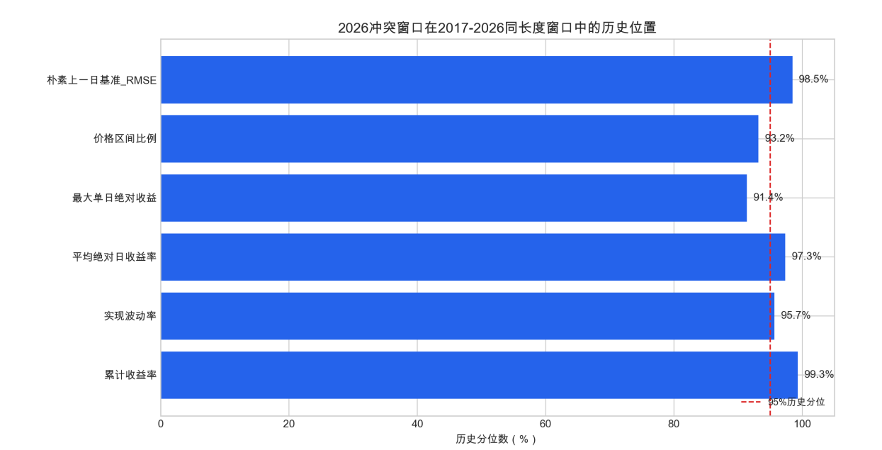
图 31 2026 冲突窗口在历史同长度窗口中的极端性。累计涨幅、波动率和朴素基准误差均处于历史高分位。
