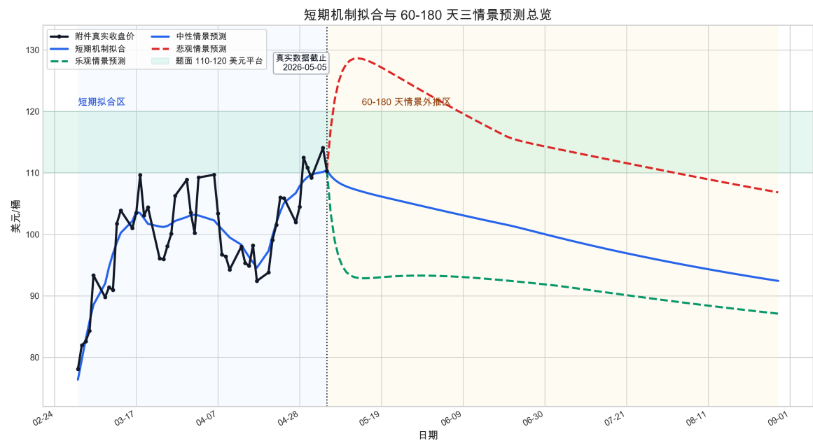
图 16: 短期机制拟合与 60–180 天三情景预测总览。竖线左侧为附件真实数据与短期模型拟合，竖线右侧为情景外推，不作为真实观测。
