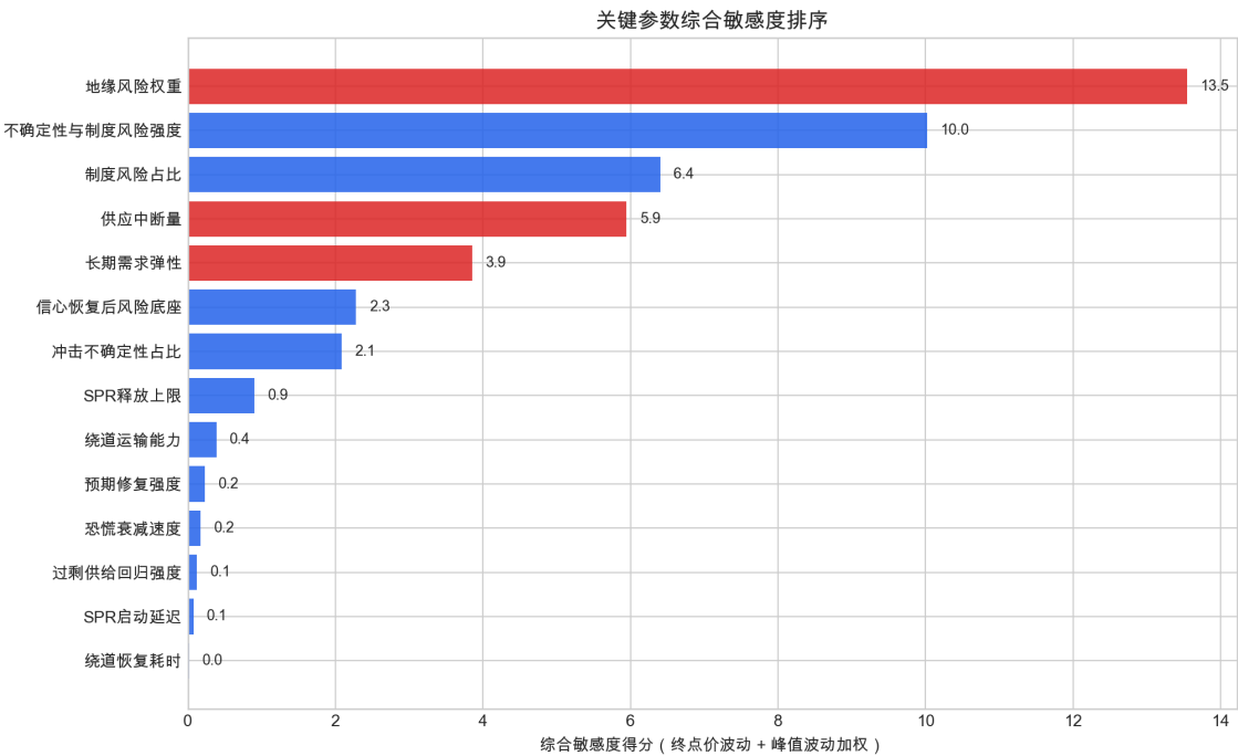
图 18: 关键参数综合敏感度排序。
