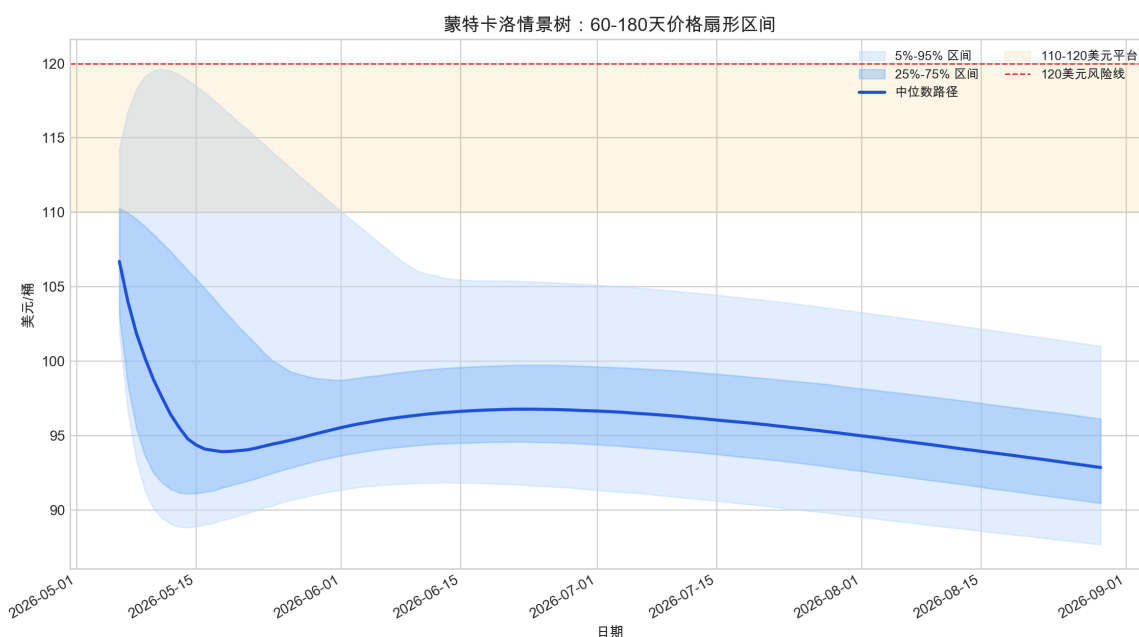
图 19: 蒙特卡洛情景树价格扇形区间。深色区间为 25%–75%，浅色区间为 5%–95%。
