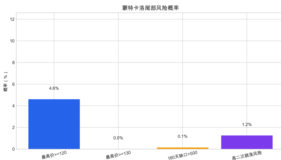
图 20: 蒙特卡洛尾部风险概率。
