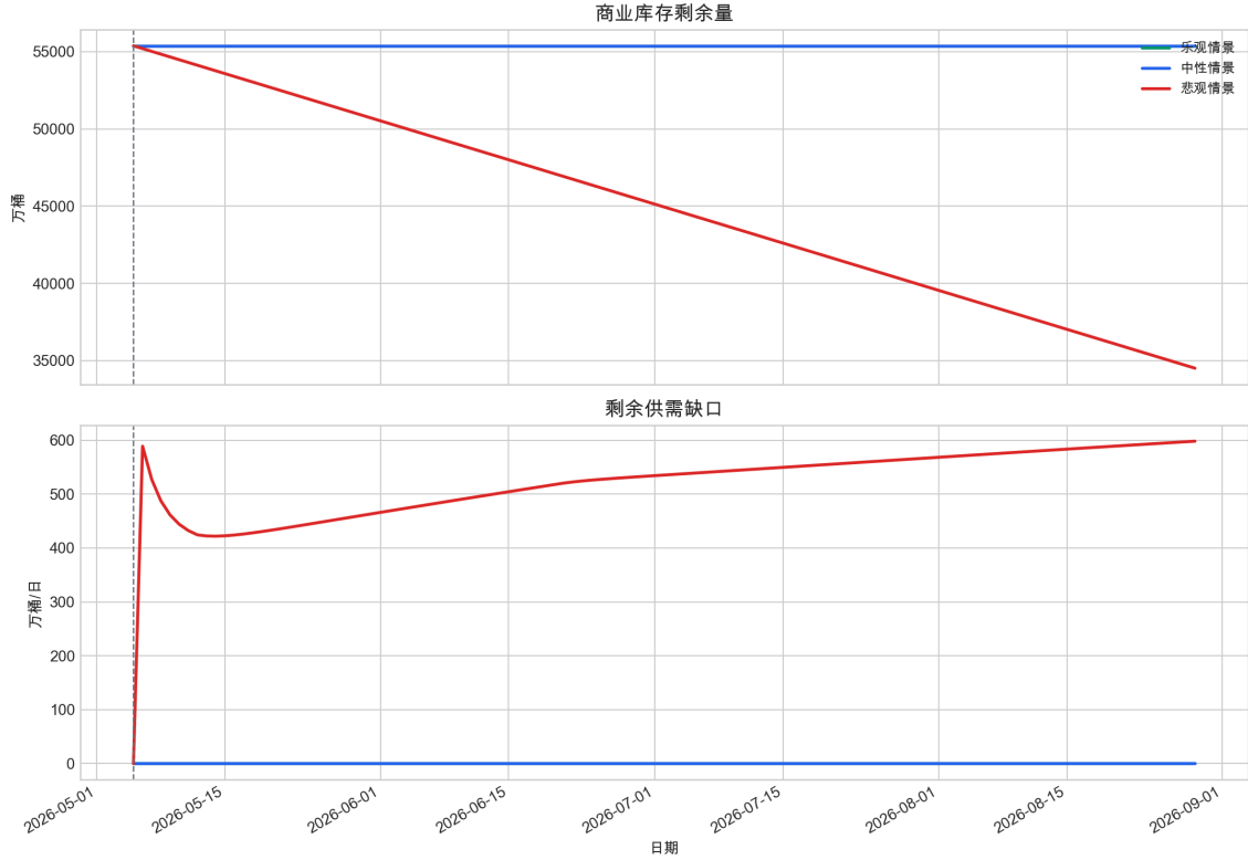
图 17: 商业库存剩余量与剩余供需缺口变化。悲观情景下缓冲能力下降，二次跳涨风险上升。
