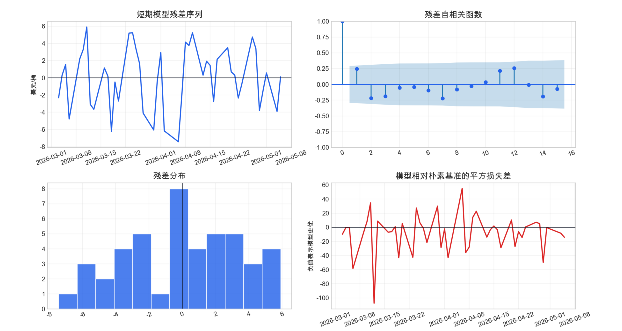
图 13: 短期模型统计审计。图中展示残差序列、残差自相关、残差分布和相对朴素基准的平方损失差。
