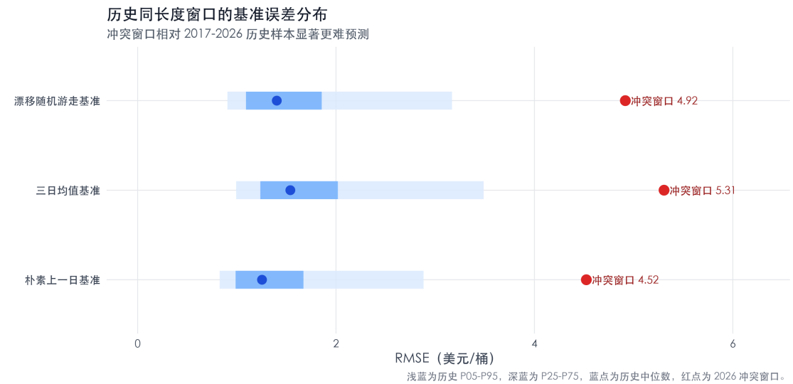
图 33 R/ggplot2 历史同长度窗口基准误差分布。蓝色区间表示历史分位带，红点表示 2026 冲突窗口，说明该窗口对普通基准模型显著更难。
