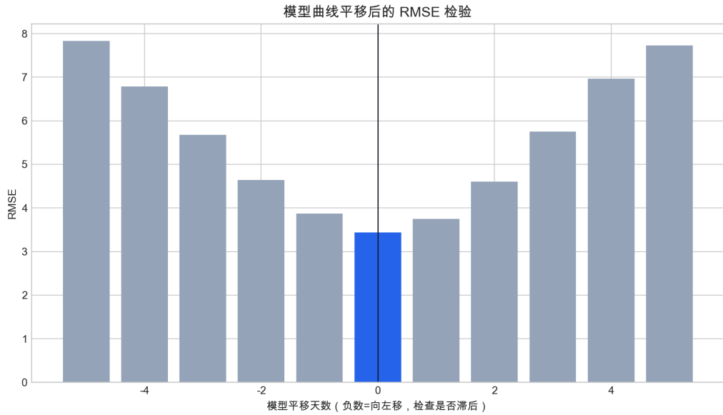
图 11 模型曲线平移后的 RMSE 检验。原始位置误差最低，说明拟合曲线不是简单把昨日真实价格滞后搬到今日。
