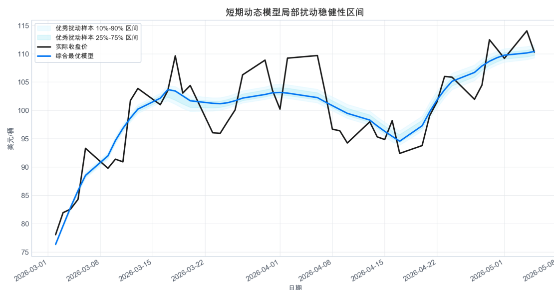
图 24 短期模型局部扰动稳健性区间。青蓝区间表示优秀扰动样本的价格分布，深蓝线为综合最优模型，黑线为实际收盘价。
