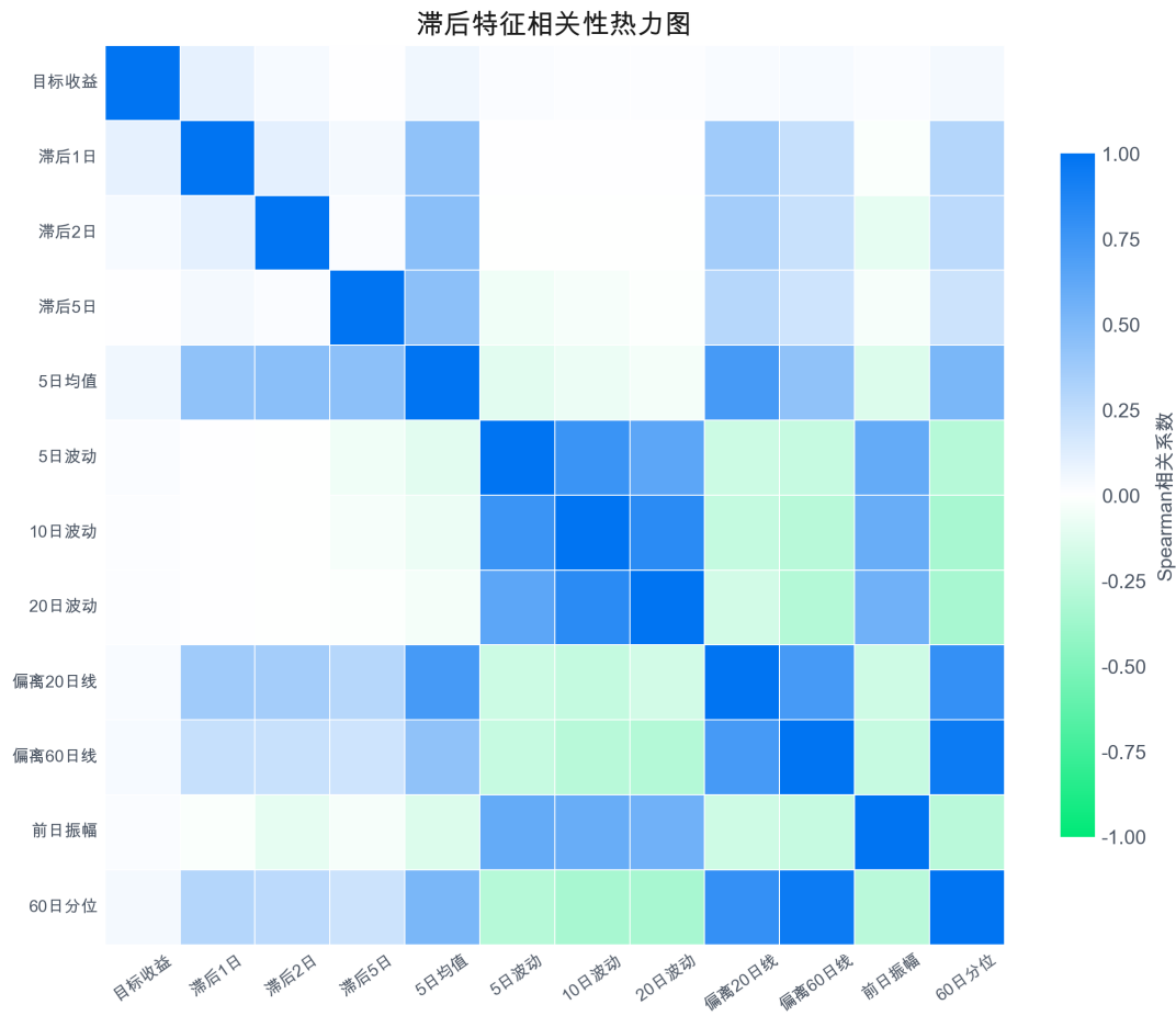
图 20 滞后价格特征相关性热力图。该图只使用目标日前可观测的历史价格特征，展示收益率、波动率、均线偏离和价格分位之间的相关结构；高相关块说明机器学习层存在信息冗余，因此本文采用低自由度 Ridge 辅助修正，而不把复杂机器学习模型作为主解释模型。
