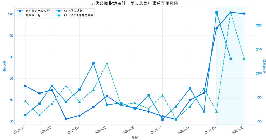
图 36 地缘风险指数检验：同步 GPR 与滞后可用 GPR。3 月油价解释不能使用 3 月同步 GPR，4 月以后才可使用已实现的 3 月风险读数。
