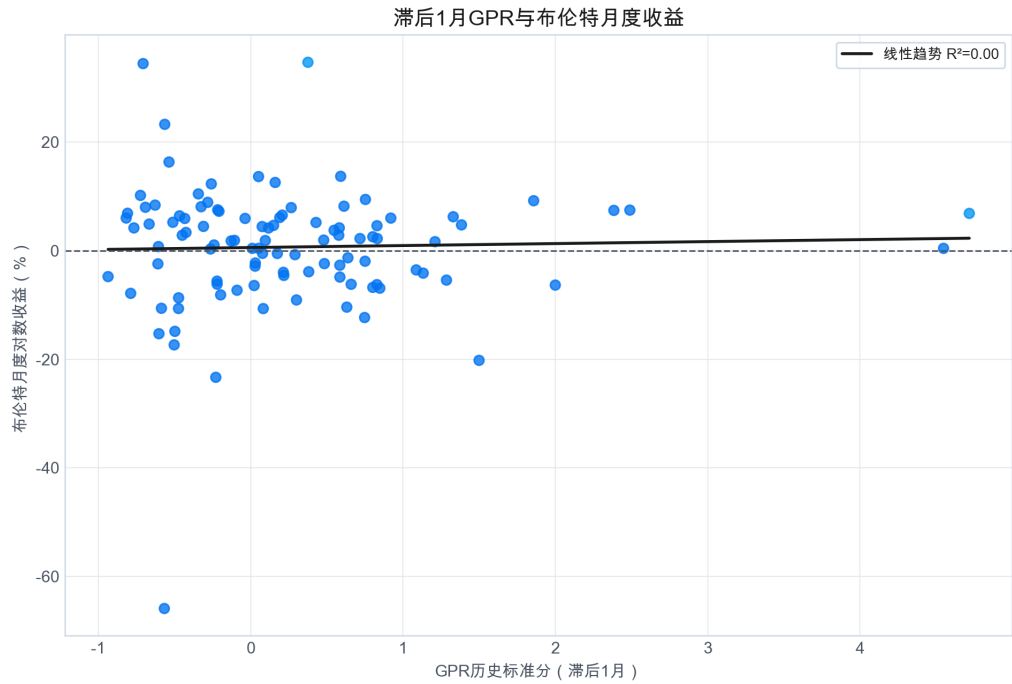
图 37 滞后 1 月 GPR 与布伦特月度收益关系。散点关系较弱，说明 GPR 更适合作为风险溢价外部校验，而非单独点预测模型。
