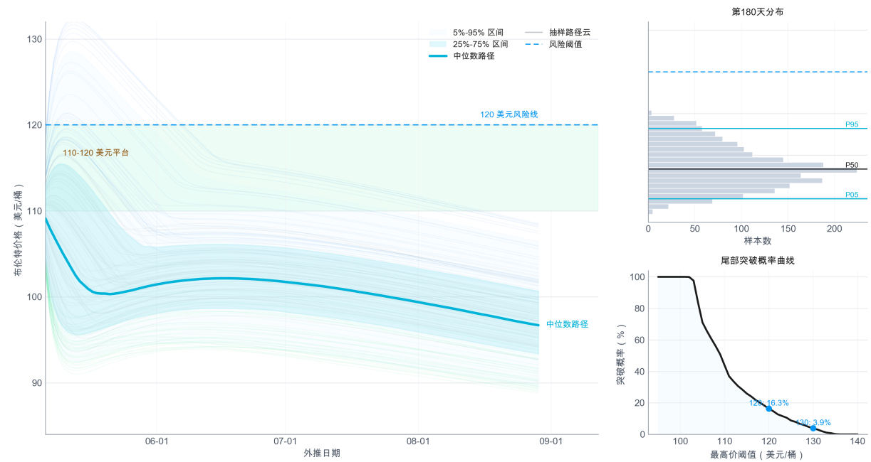
图 26 长期情景预测主图：蒙特卡洛情景树高级组合图。左侧展示中心路径、抽样路径云和 5%–95% / 25%–75% 条件区间，右上展示第 180 天终点分布，右下展示外推期突破 120、130 美元/桶的累计概率曲线；该图证明长期结论应读作条件区间和尾部概率，而不是单点预测。
