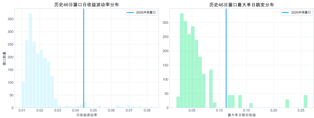
图 32 历史波动参数校准。2017–2025 同长度窗口为长期蒙特卡洛和状态转移扰动提供历史尺度。
