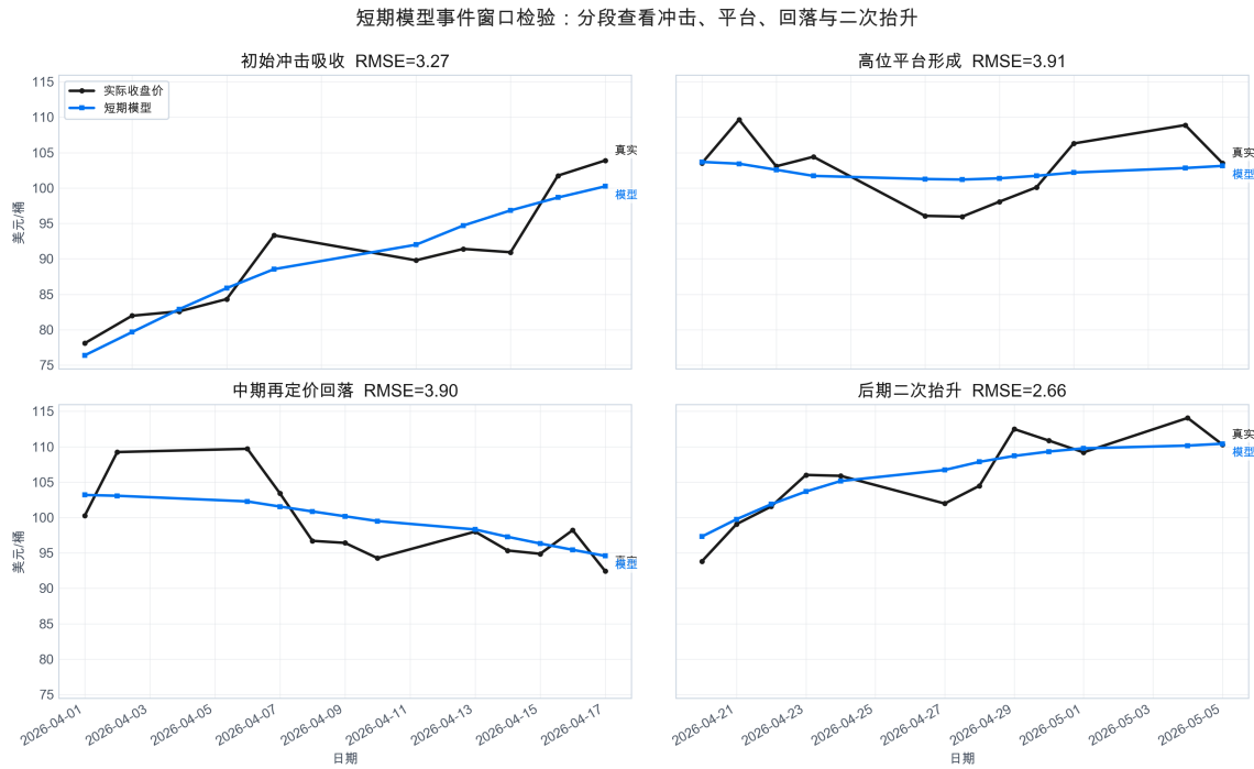
图 22 短期模型事件窗口检验。该图将总拟合曲线拆成四个关键事件段，显示模型在初始冲击和后期抬升段拟合较稳，在高位平台与中期回落段仍面临更高日度噪声。
