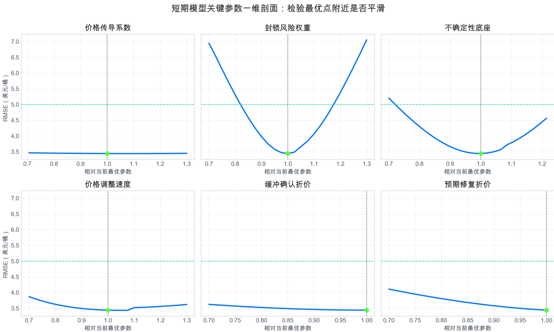
图 23 短期模型关键参数一维剖面。横轴为相对当前最优参数的比例，绿点为当前参数位置，虚线为 RMSE=5 的稳健性参考阈值；图中曲线用于检验模型是否依赖孤立参数点。
