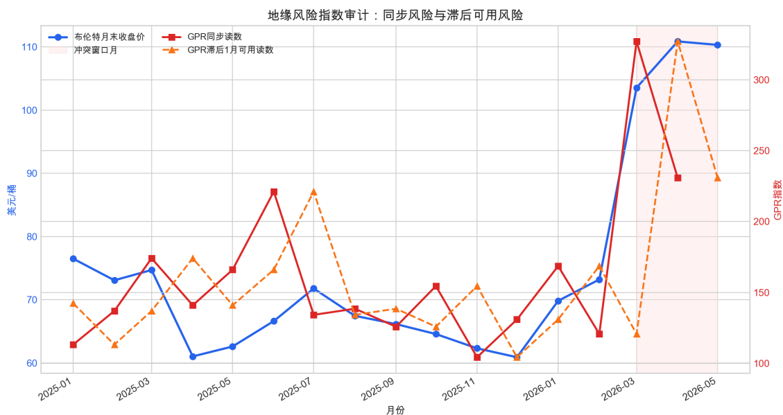
图 25 地缘风险指数审计：同步 GPR 与滞后可用 GPR。3 月油价解释不能使用 3 月同步 GPR，4 月以后才可使用已实现的 3 月风险读数。
