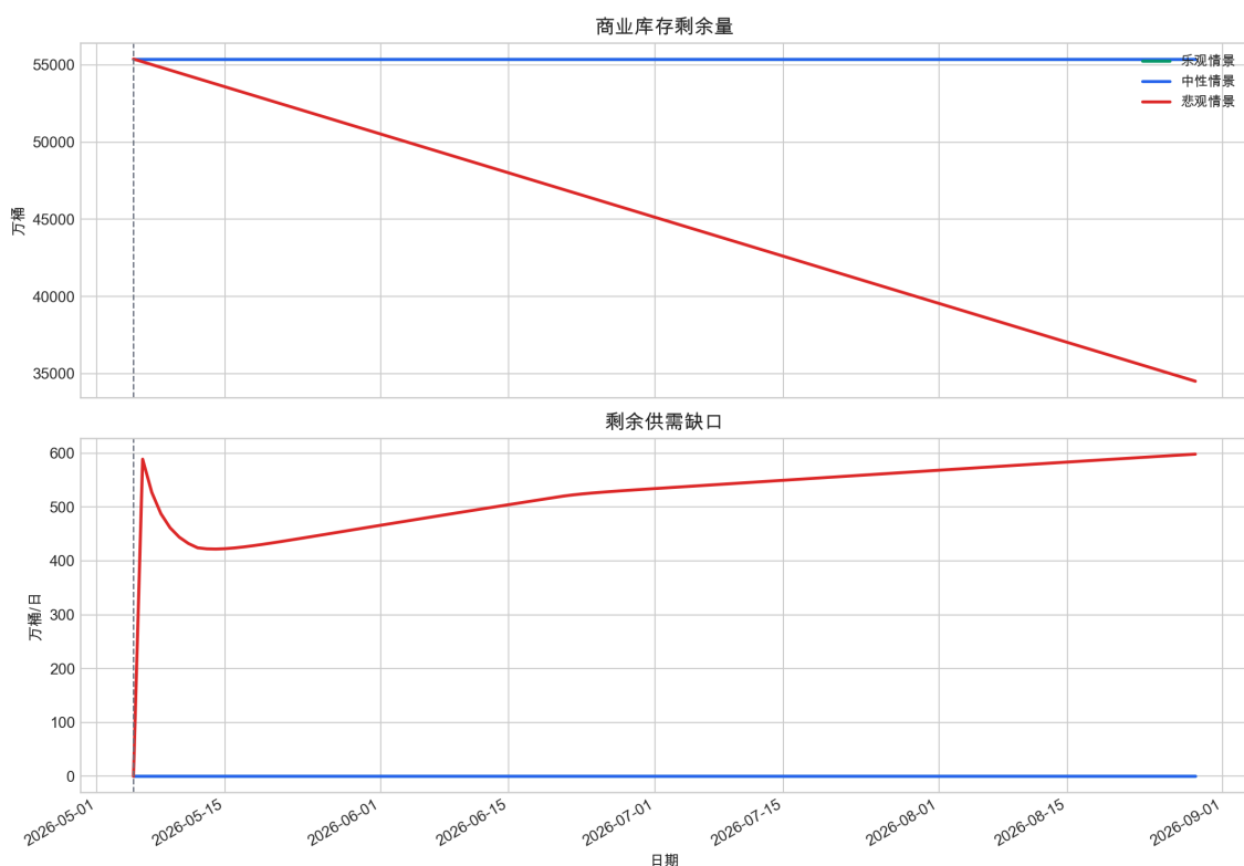
图 21 商业库存剩余量与剩余供需缺口变化。悲观情景下缓冲能力下降，二次跳涨风险上升。
