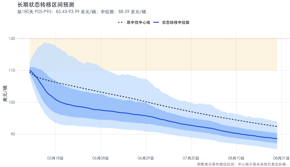
图 24 R/ggplot2 长期状态转移区间预测。双层阴影分别表示 5%–95% 和 25%–75% 条件区间，虚线为原中性中心路径。
