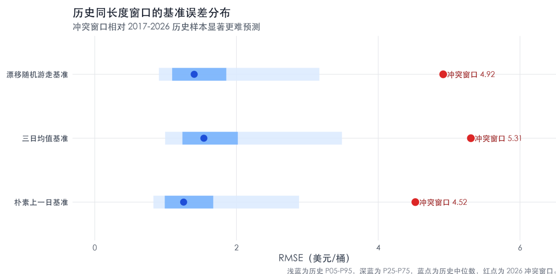
图 28 R/ggplot2 历史同长度窗口基准误差分布。蓝色区间表示历史分位带，红点表示 2026 冲突窗口，说明该窗口对普通基准模型显著更难。
