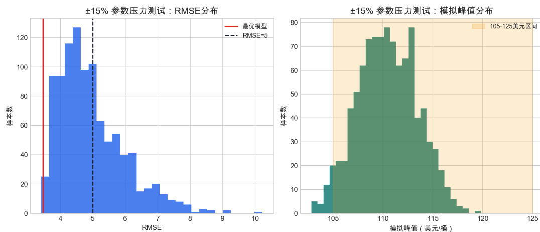
图 12 短期模型过拟合压力测试。多数扰动样本仍保持在合理价格平台附近。
