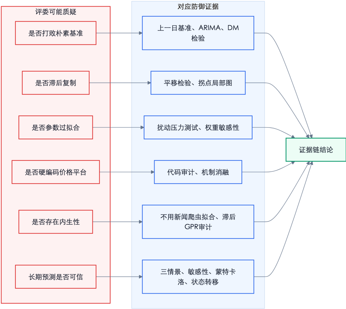
图 9 评审质疑防御框架。每类潜在质疑都对应可复现的检验、图表或审计输出。
